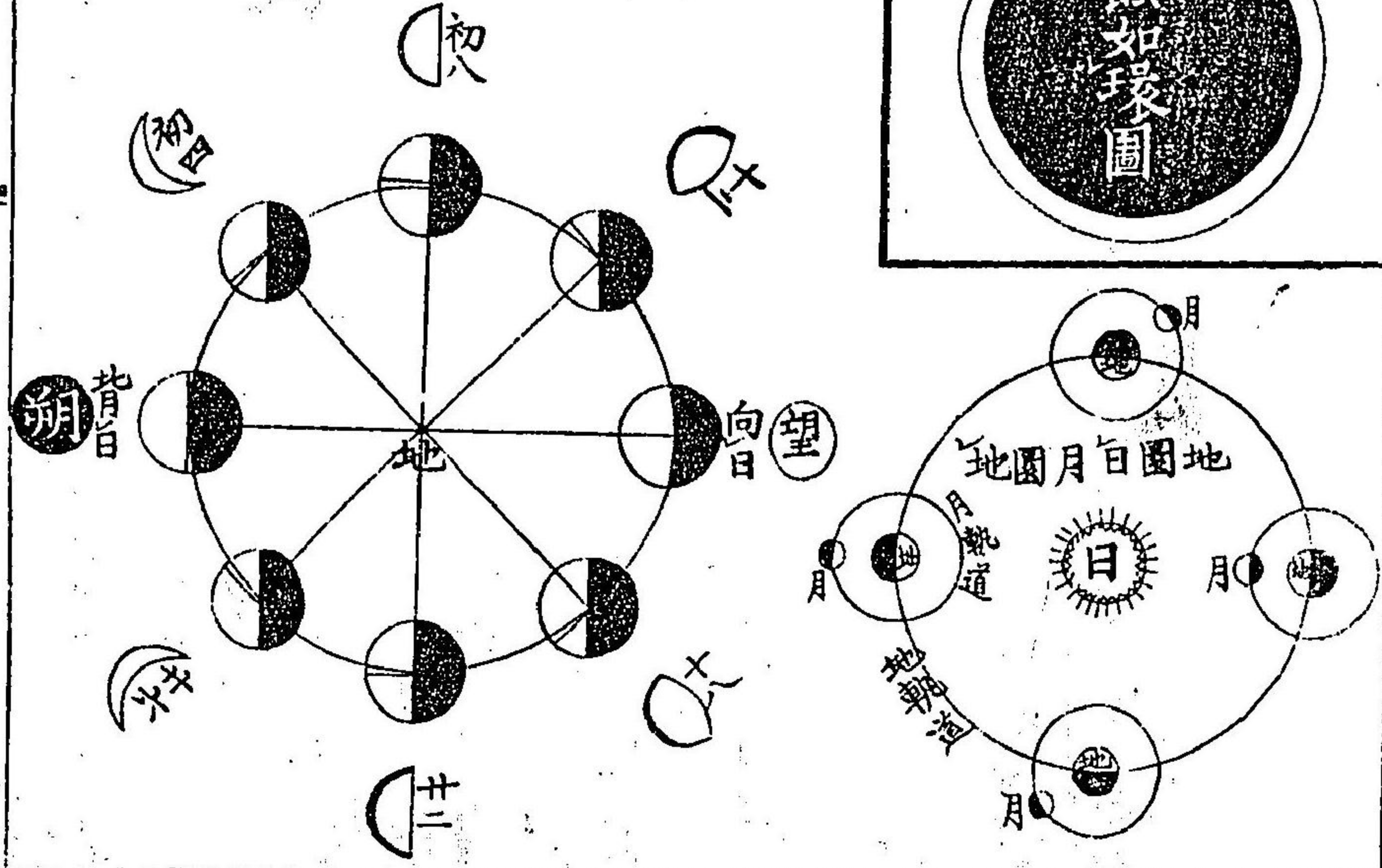
圖望朔成地圓輪月
