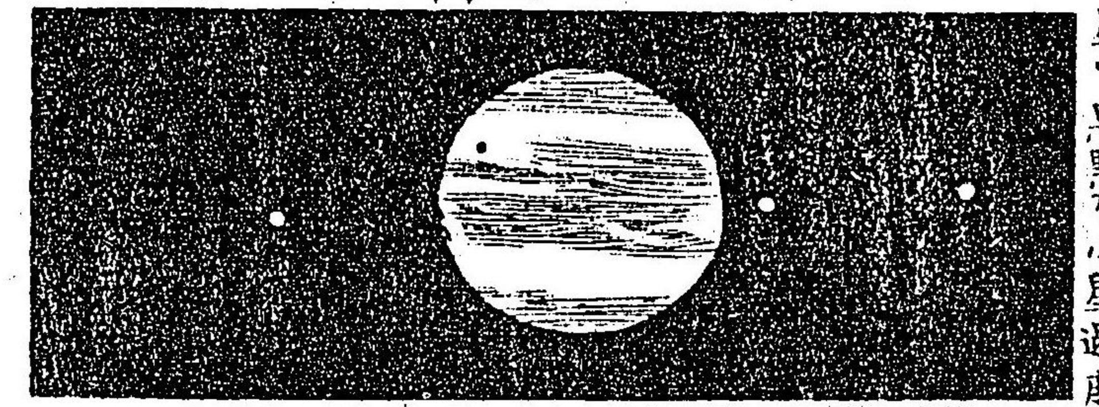
木星形體及四小行星之圖
