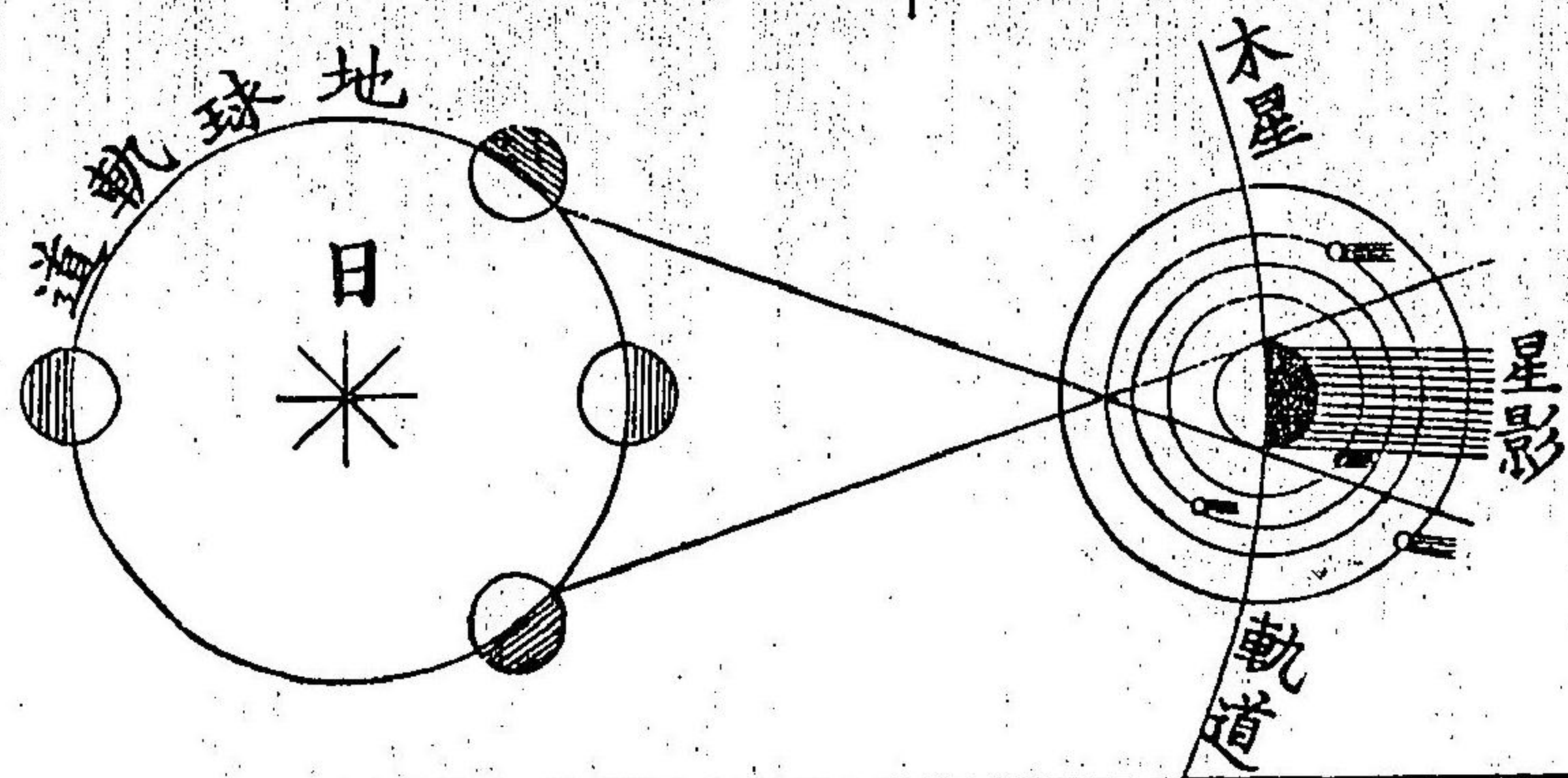
四星小行星行木之星圖
