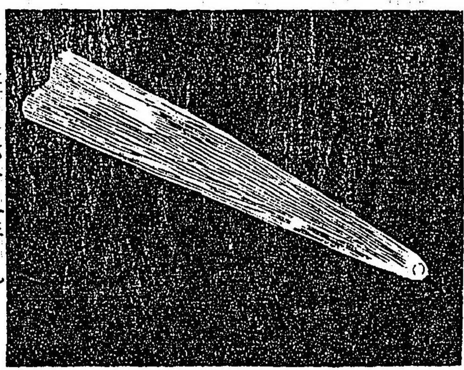
彗星之圖
