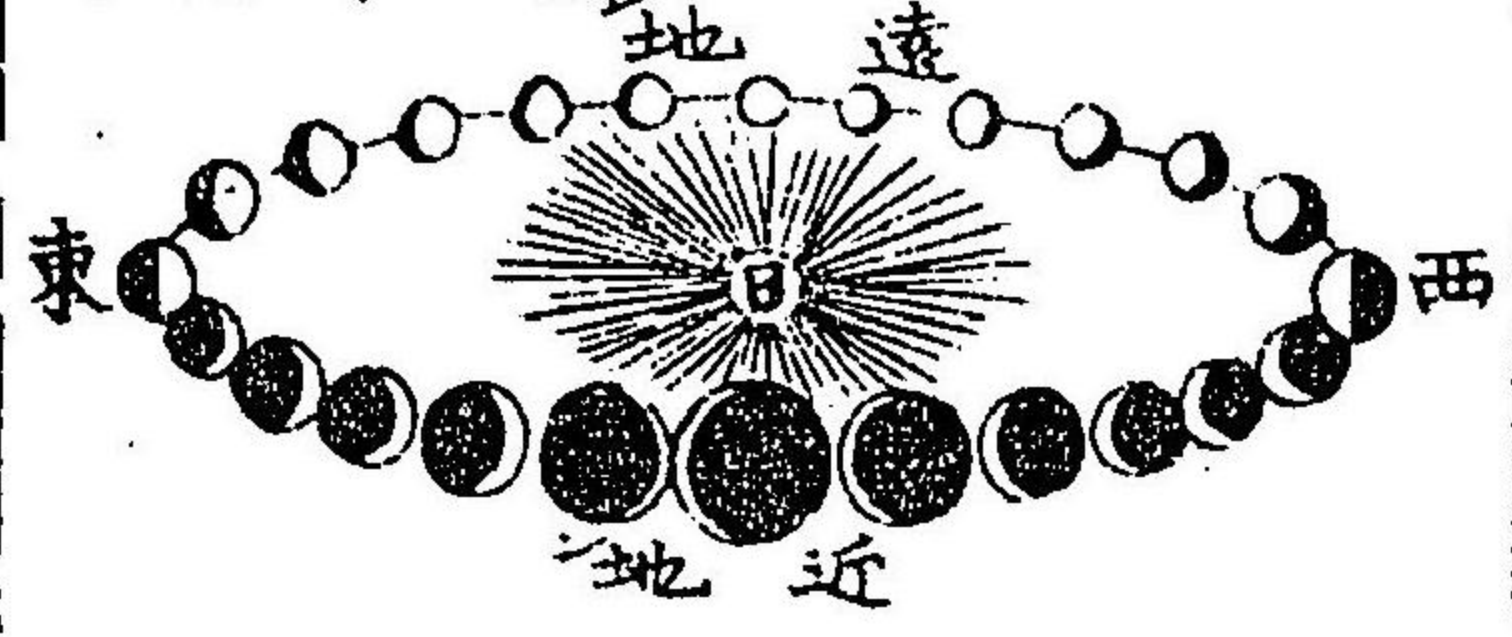
金星圍日成盈缺之圖
