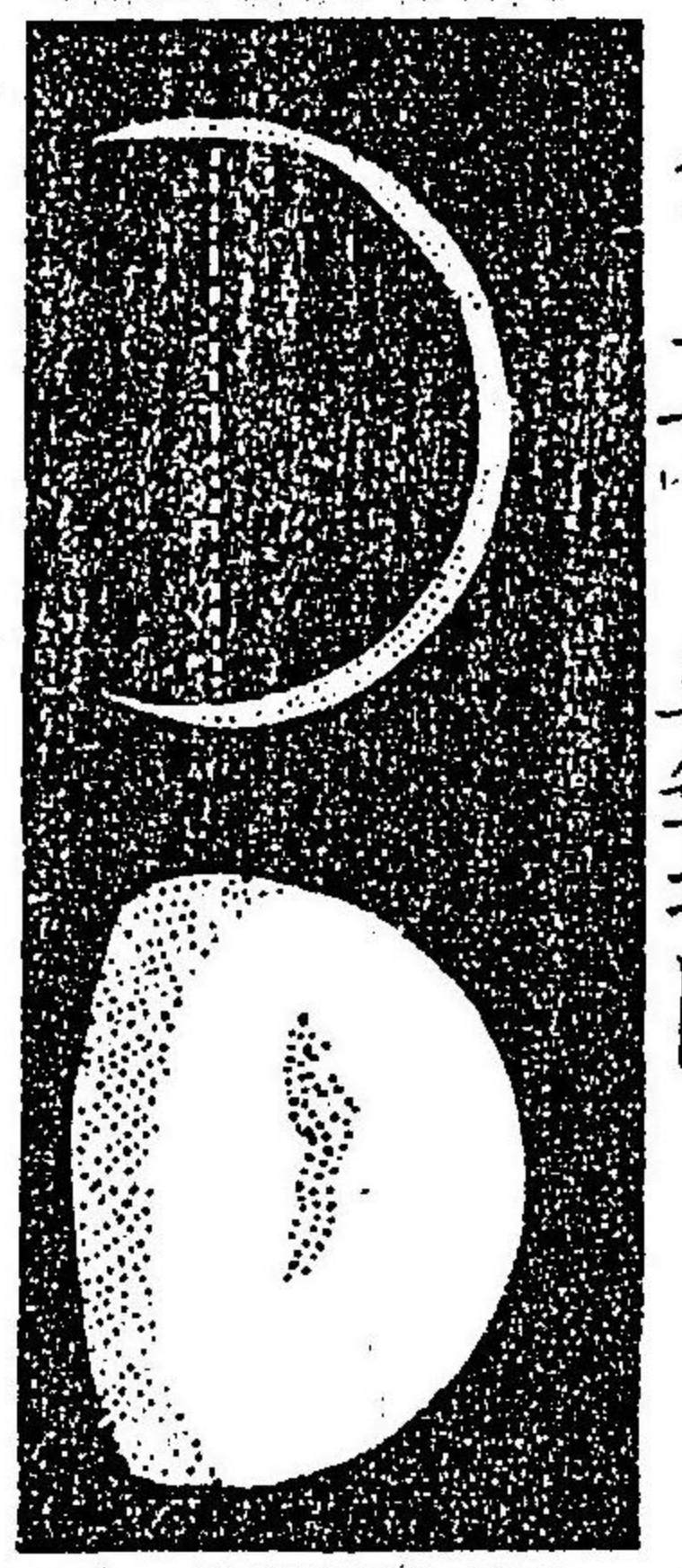
火星將盈之圖
