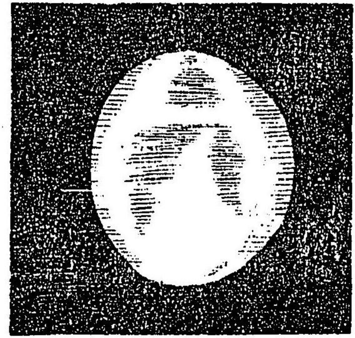
火星將盈之圖
