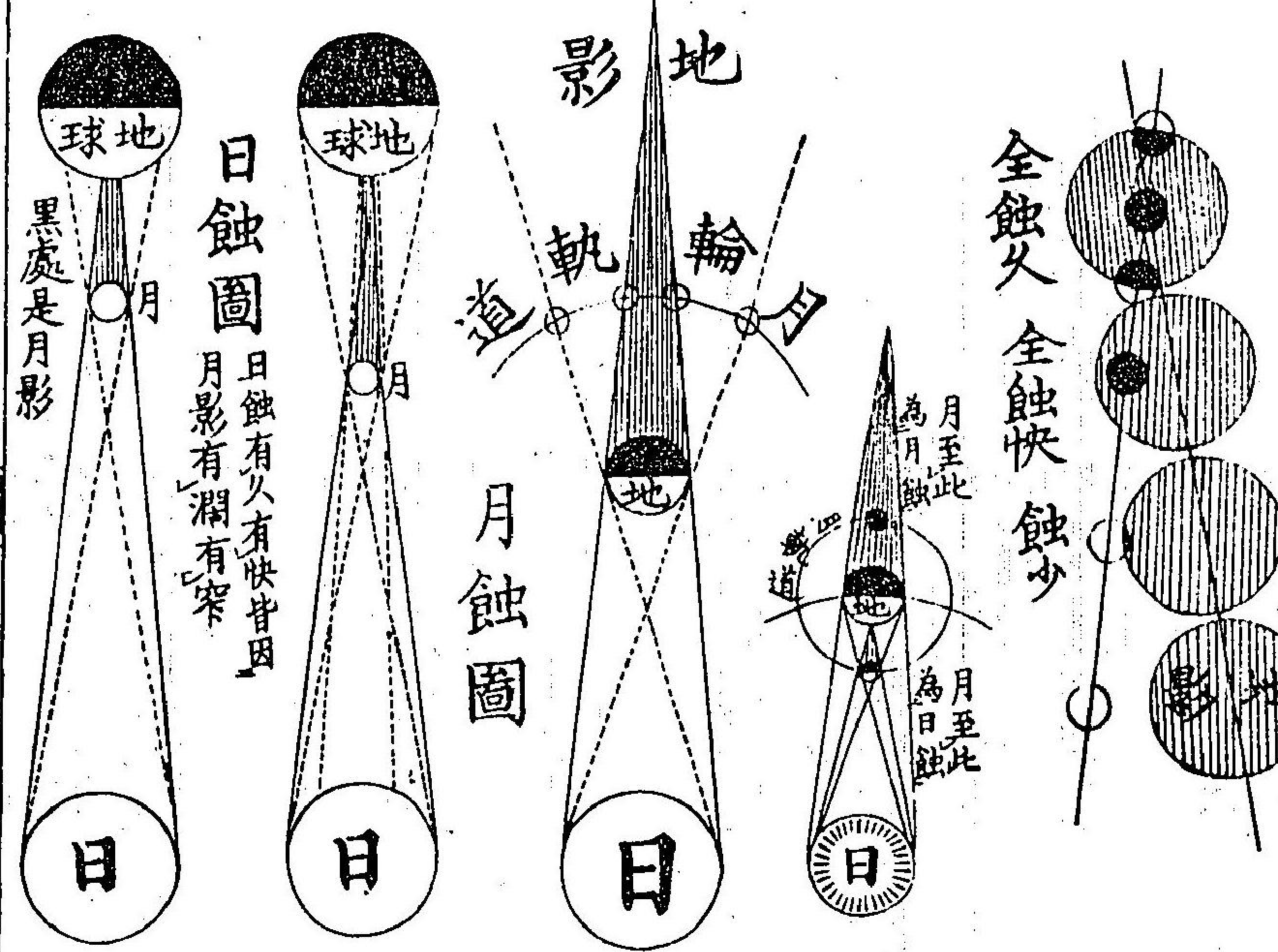
地影掩月圖
