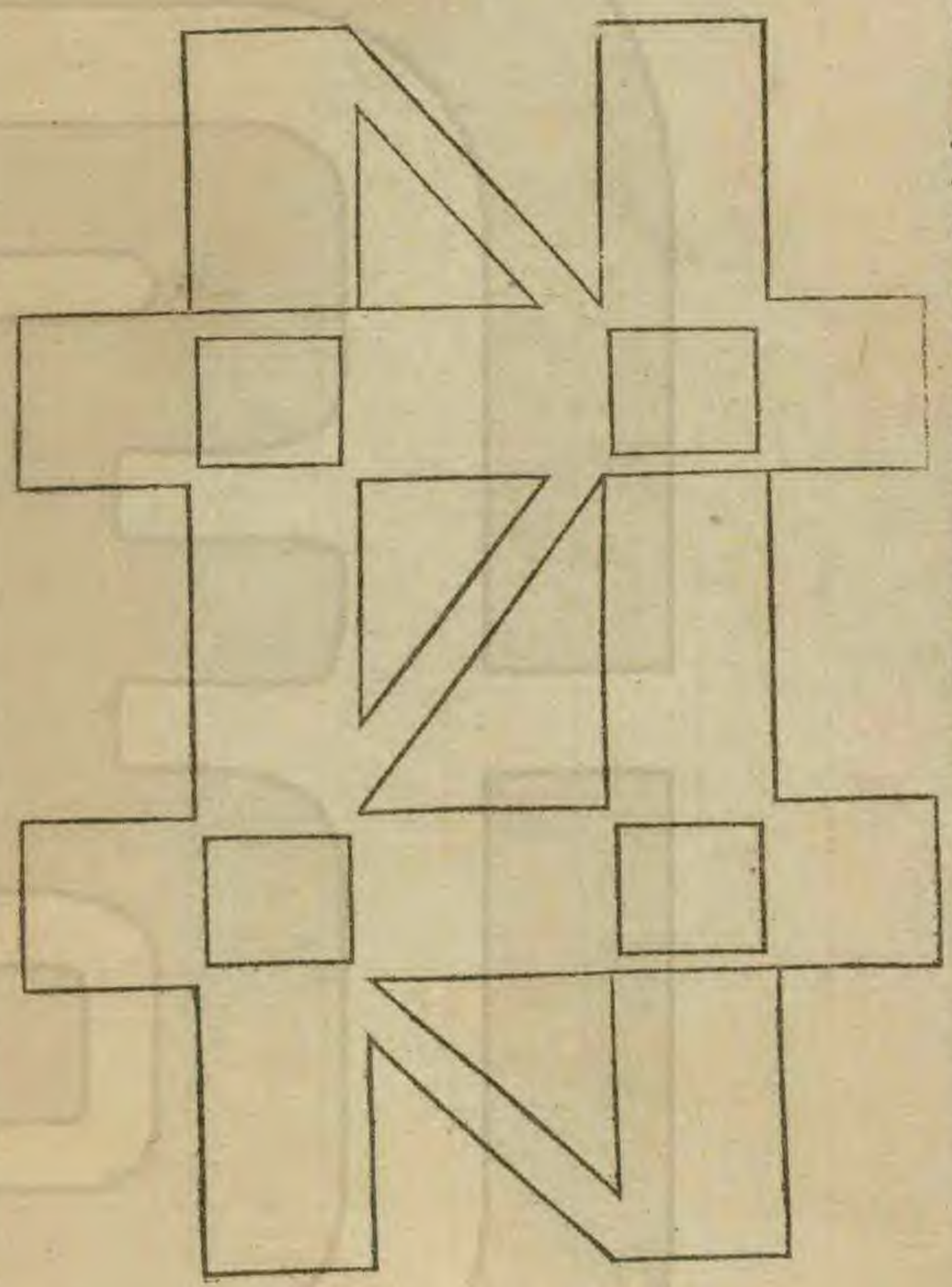
式圖溝火穀炕
