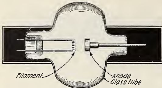
FIG. 13 Gas tube rectifier
