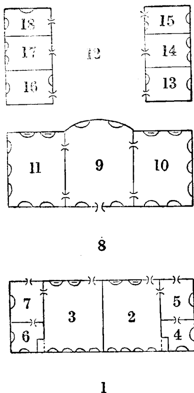
複式小學校舍平面圖
