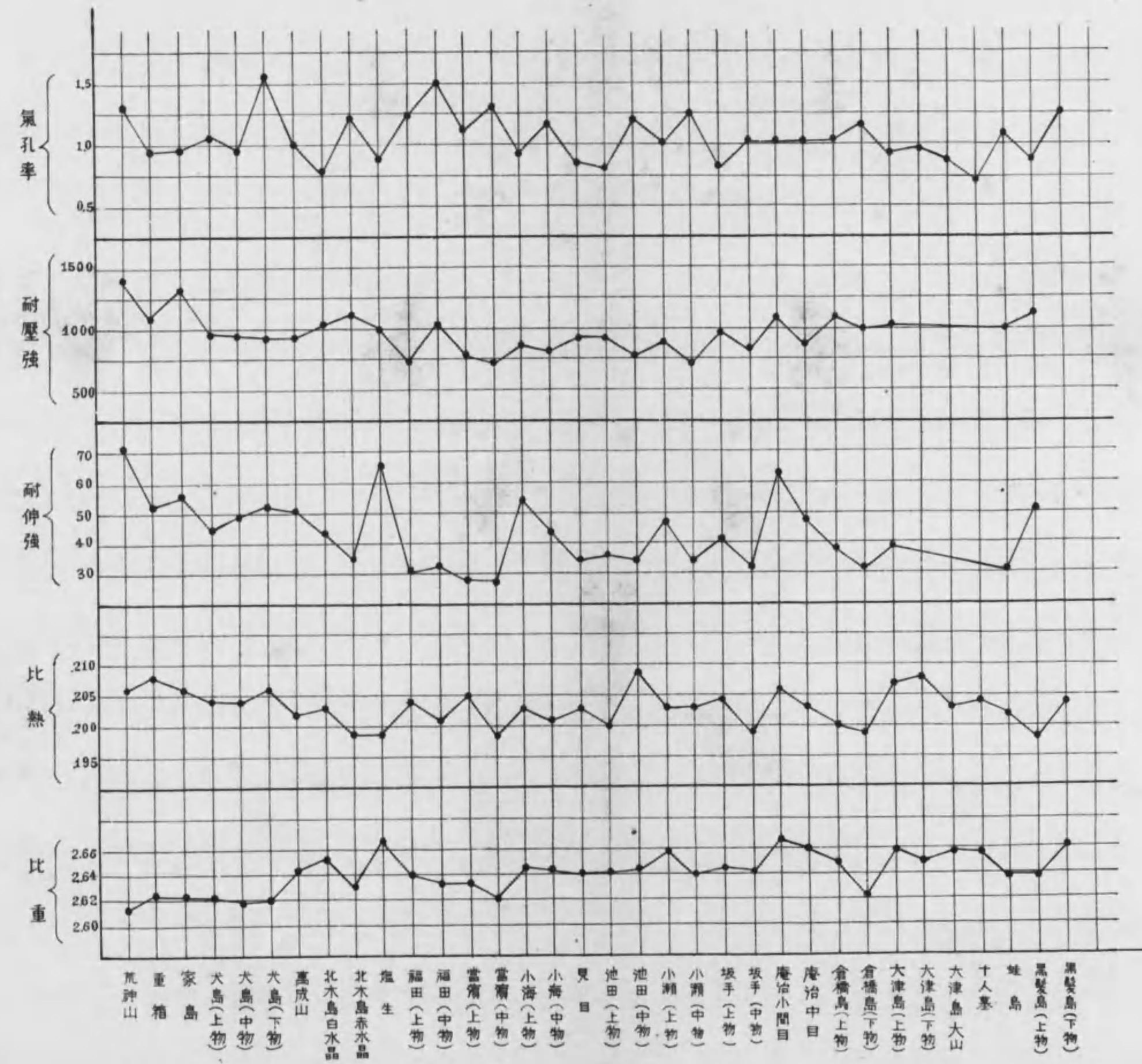
中國産花崗岩ノ比重、比熱、耐伸強、耐壓強及氣孔率ヲ表ス曲線
