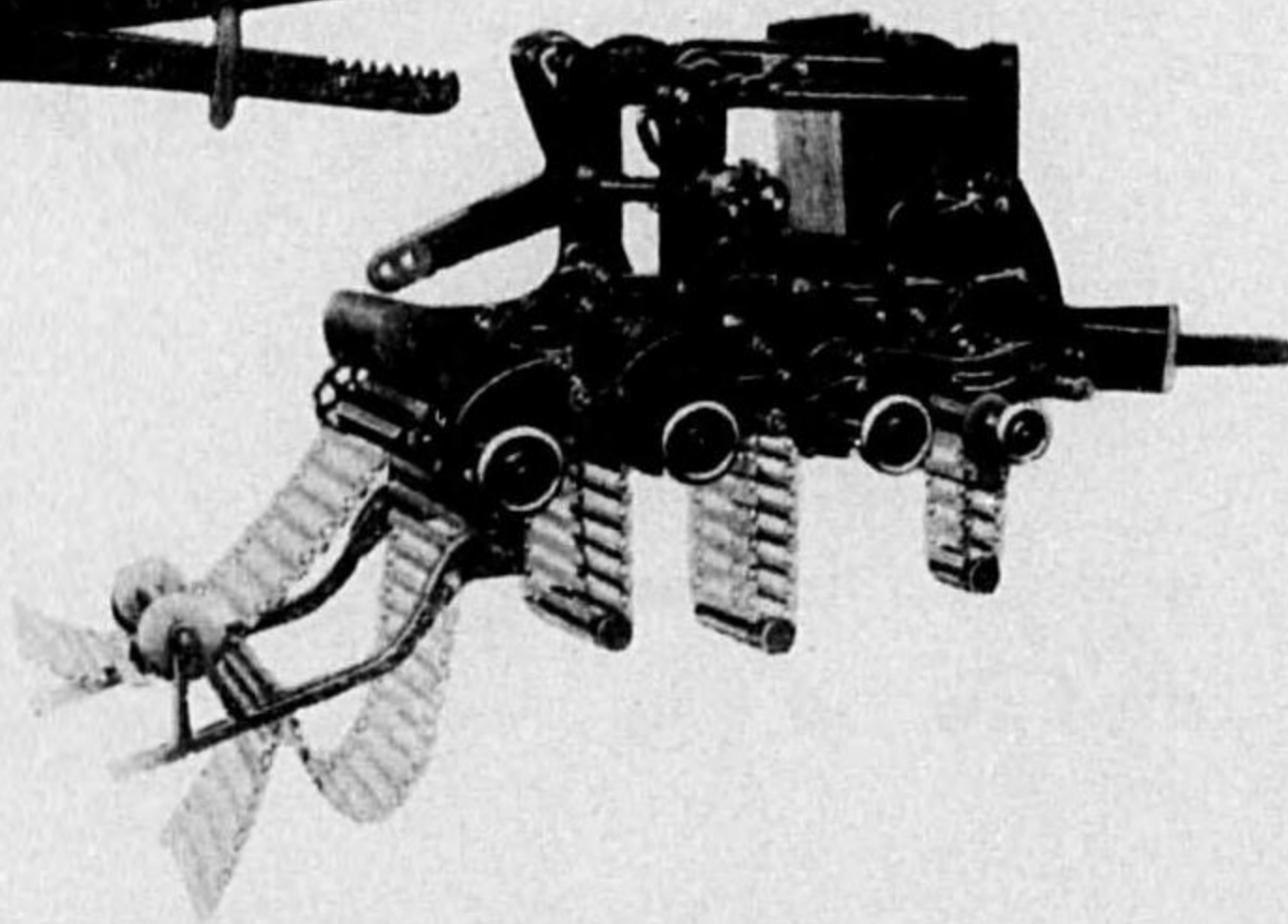
三本シリンダー ドビー装置
