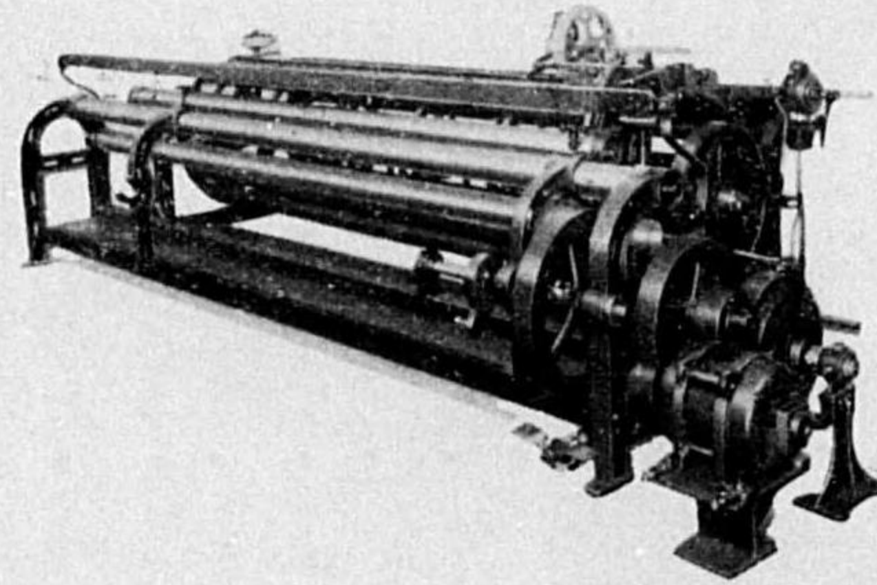
奥井式管捲機
