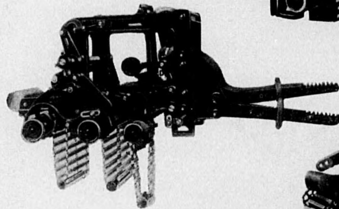
自動式Wシリンダー ドビー装置
