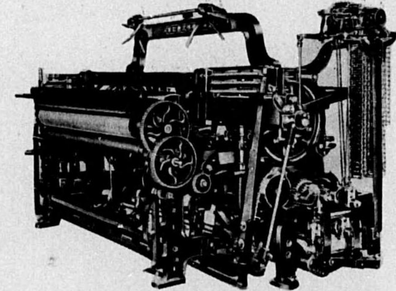
高級織物用 專賣特許阪本式 兩側四挺杼織機
