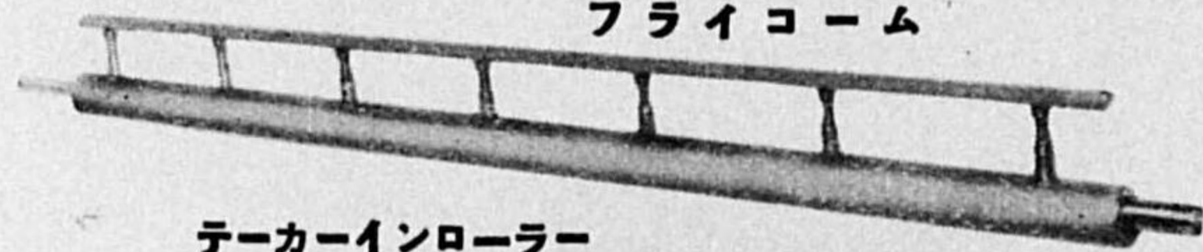
テーカーインローラー
