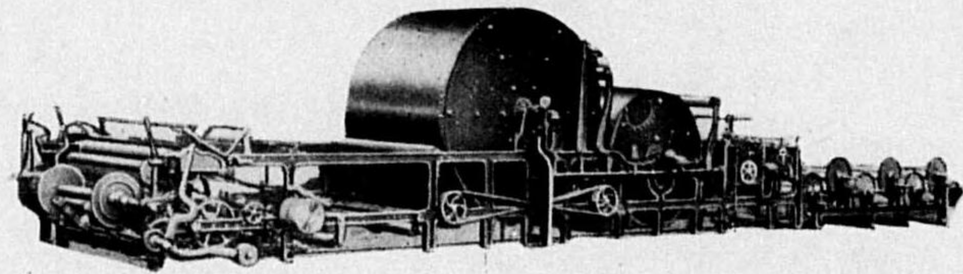
特許水平式布疊機
