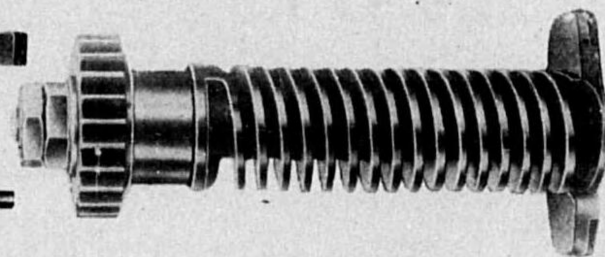
フォーラー・スクリユー
