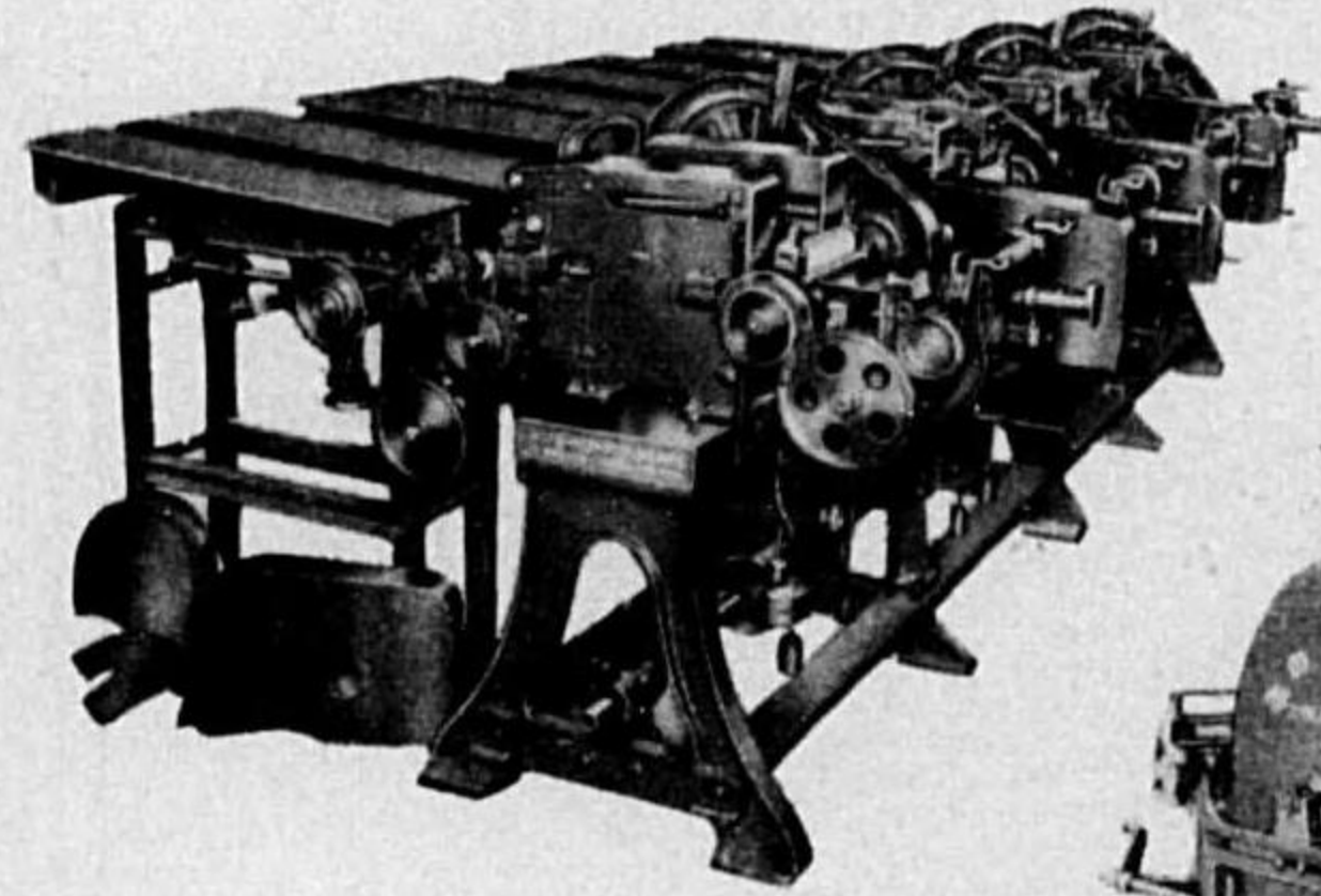
米式製襪機
