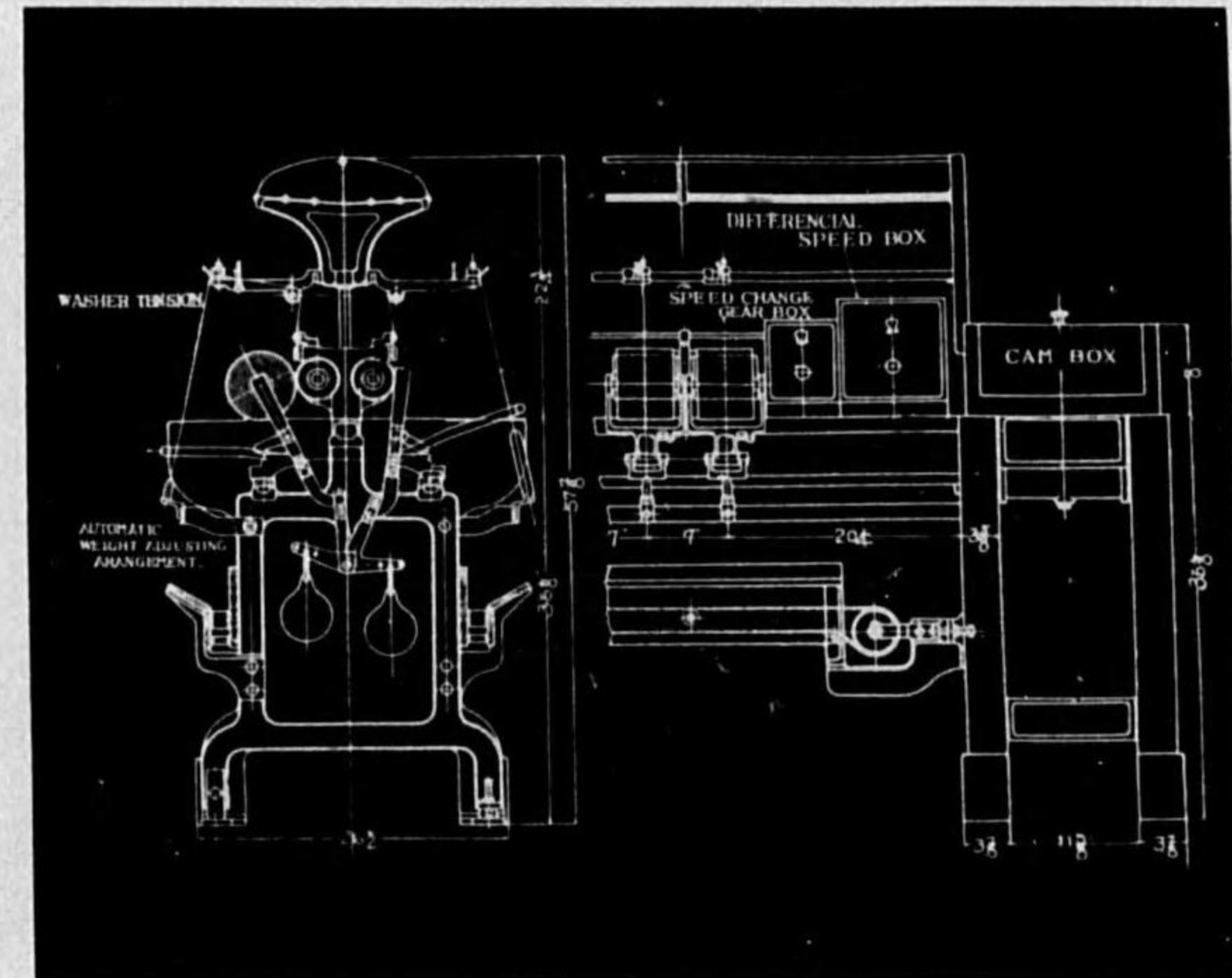
クイツク・トラバース・ワインダー セミハイスピード (特許出願中)
