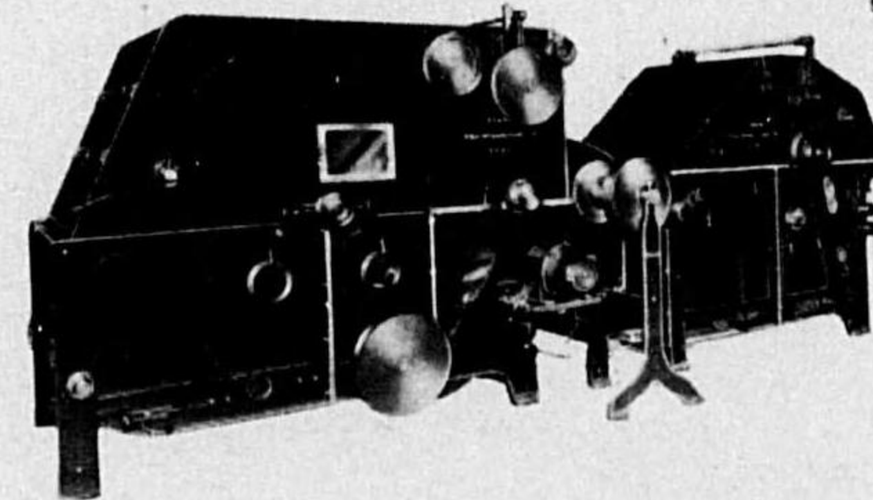
O. K. K. Hopper Bale Breaker and Hopper Feeder for Staple Fibre
