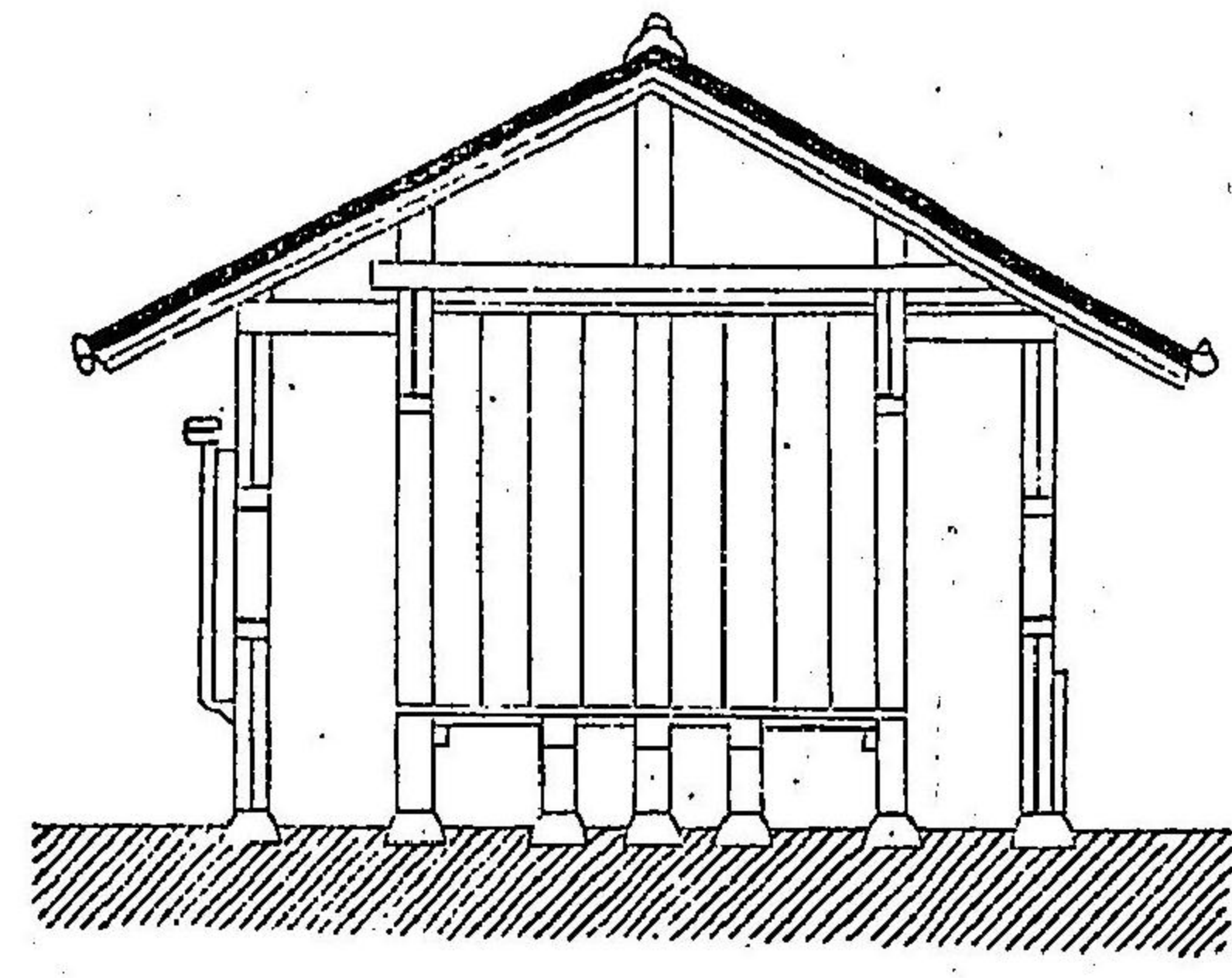
圖斷橫
