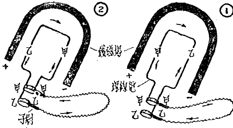
交流發電機發電原理
