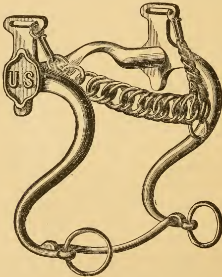
Fig. 13.—"MCCLELLAN" BIT.
