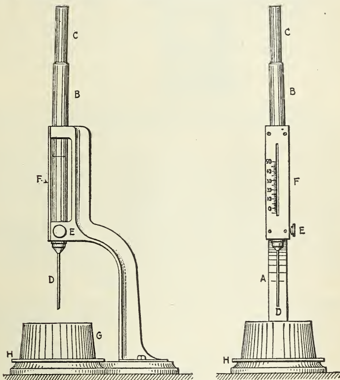
FIG. 10.—Vicat apparatus.
