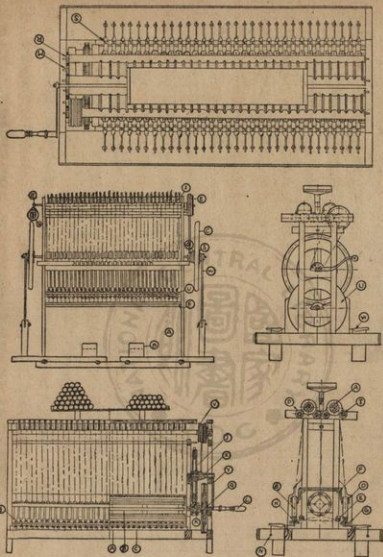
徐桃紡紗機說明圖
