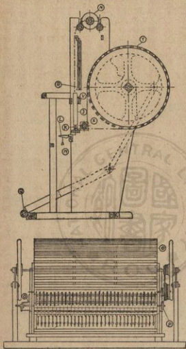
七七紡紗機說明圖
