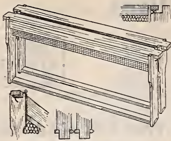
Hoffman Frame.
