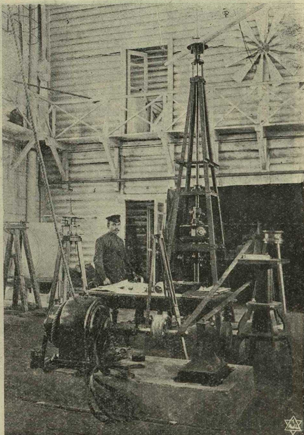
Аппаратъ для изученія винтовъ большаго діаметра.
