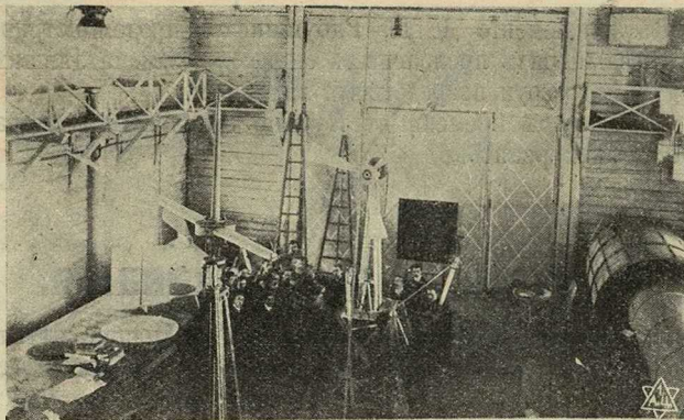
Общій видъ главнаго зала аэродинамическаго института. Слева приборъ для изученія тренія воздуха о поверхность.
