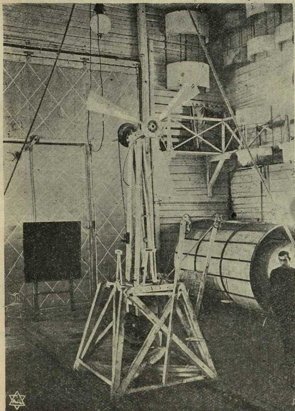
Аппаратъ Ренарда для опредѣленія тяги винта.
