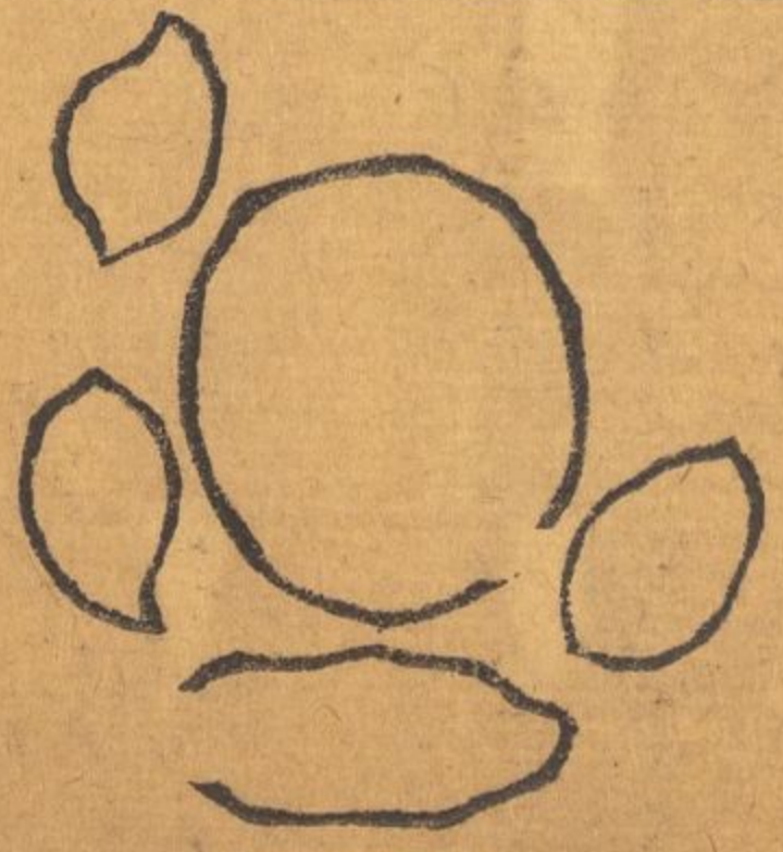
濠州銀星石
