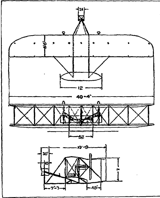
胡賴的第一個雙翼機
