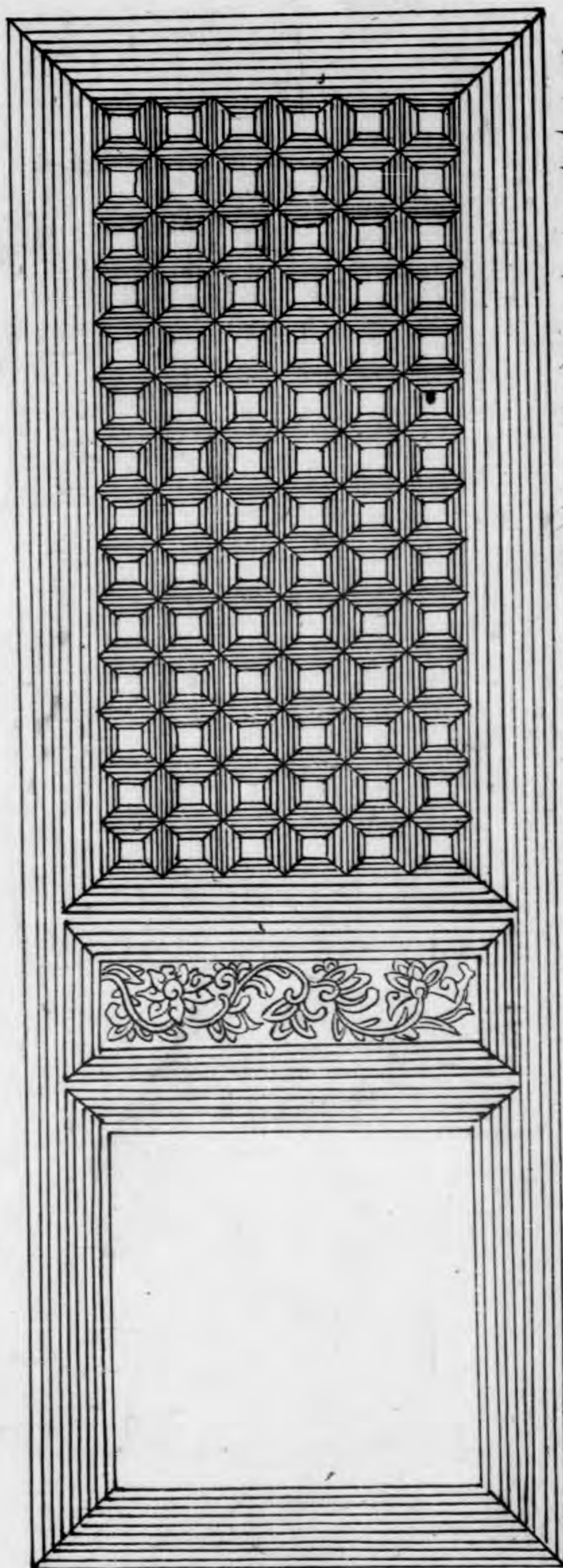
四程破瓣單混平地出單線
