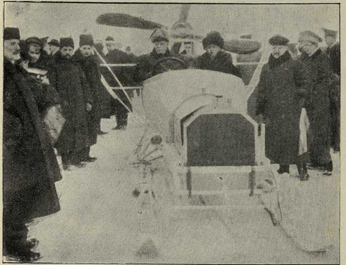
Аэро-сани Ю. А. Меллера.
