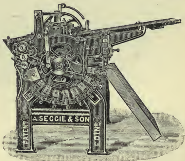
Fig. 20. BRONZING MACHINE.
