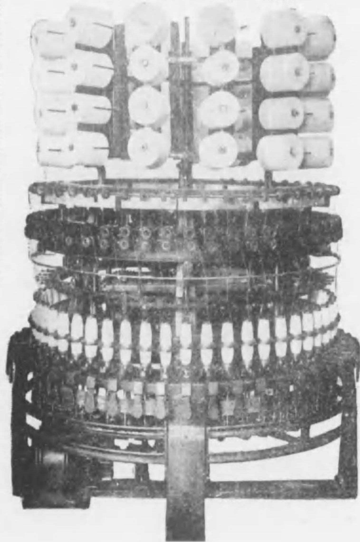
〔丸型撚糸機〕
