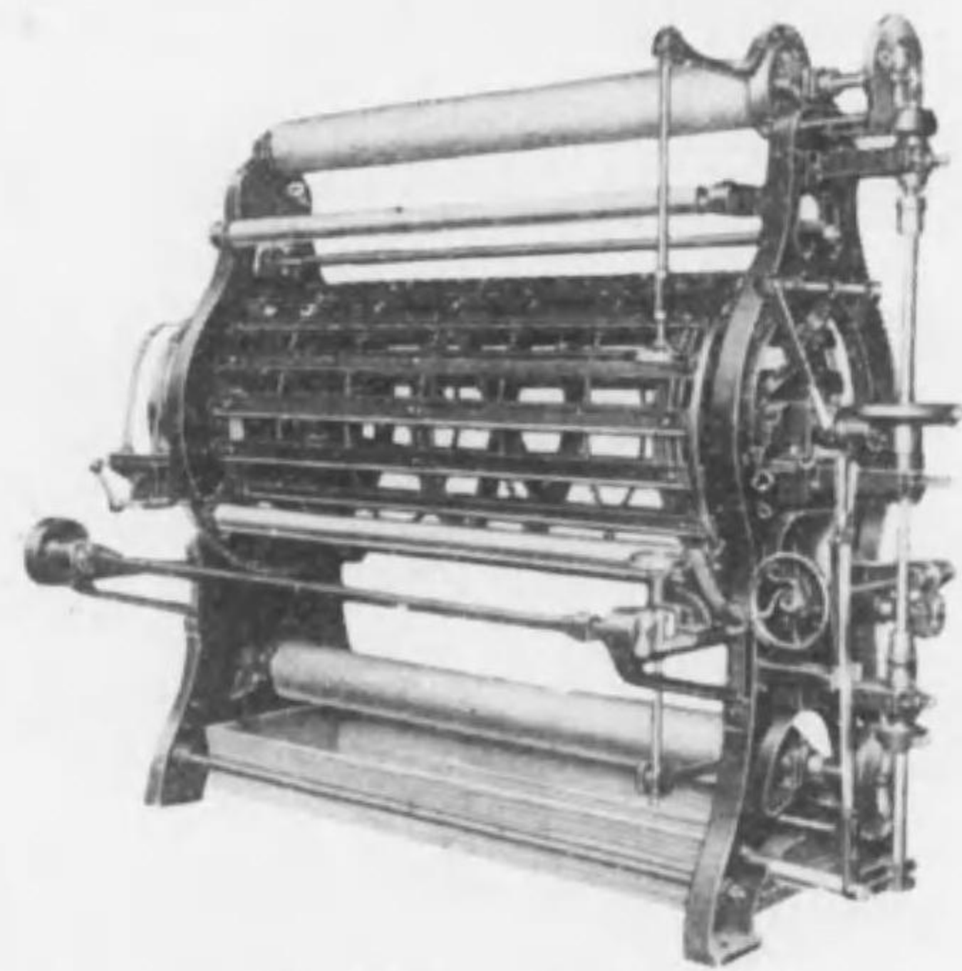
滯搔「ミザア」起毛機
