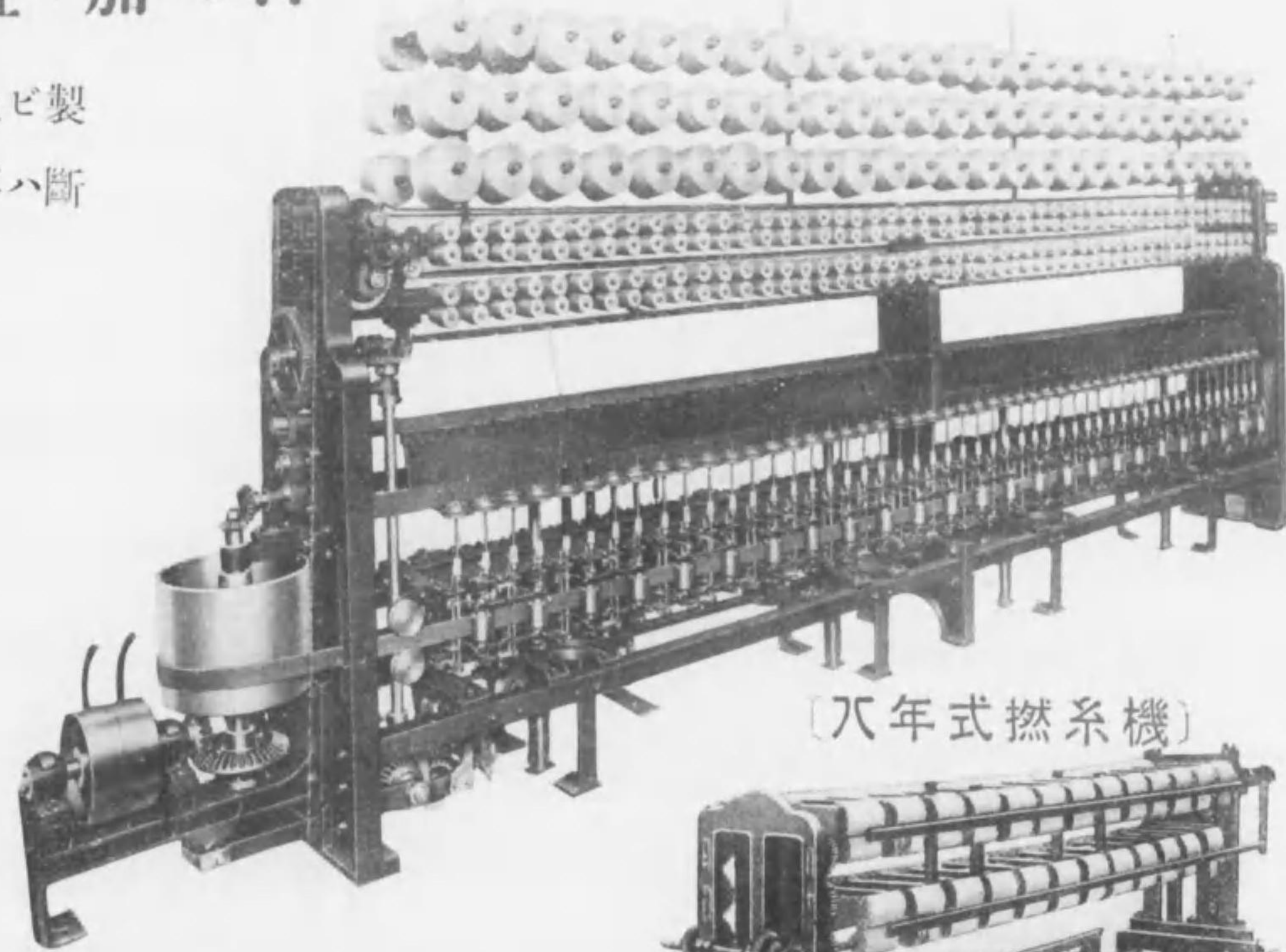
〔整動撚糸機〕
