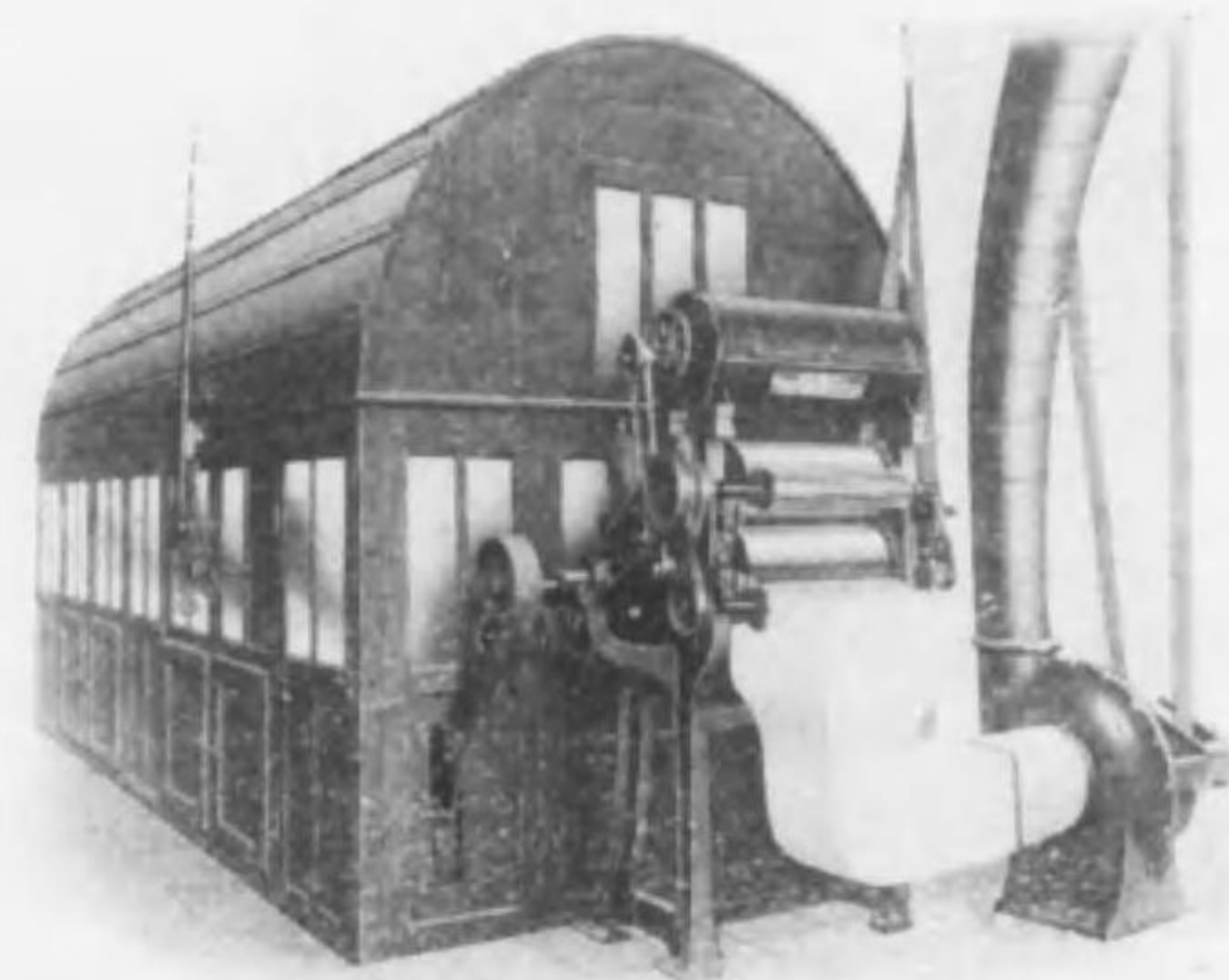
熱風式乾毛機
