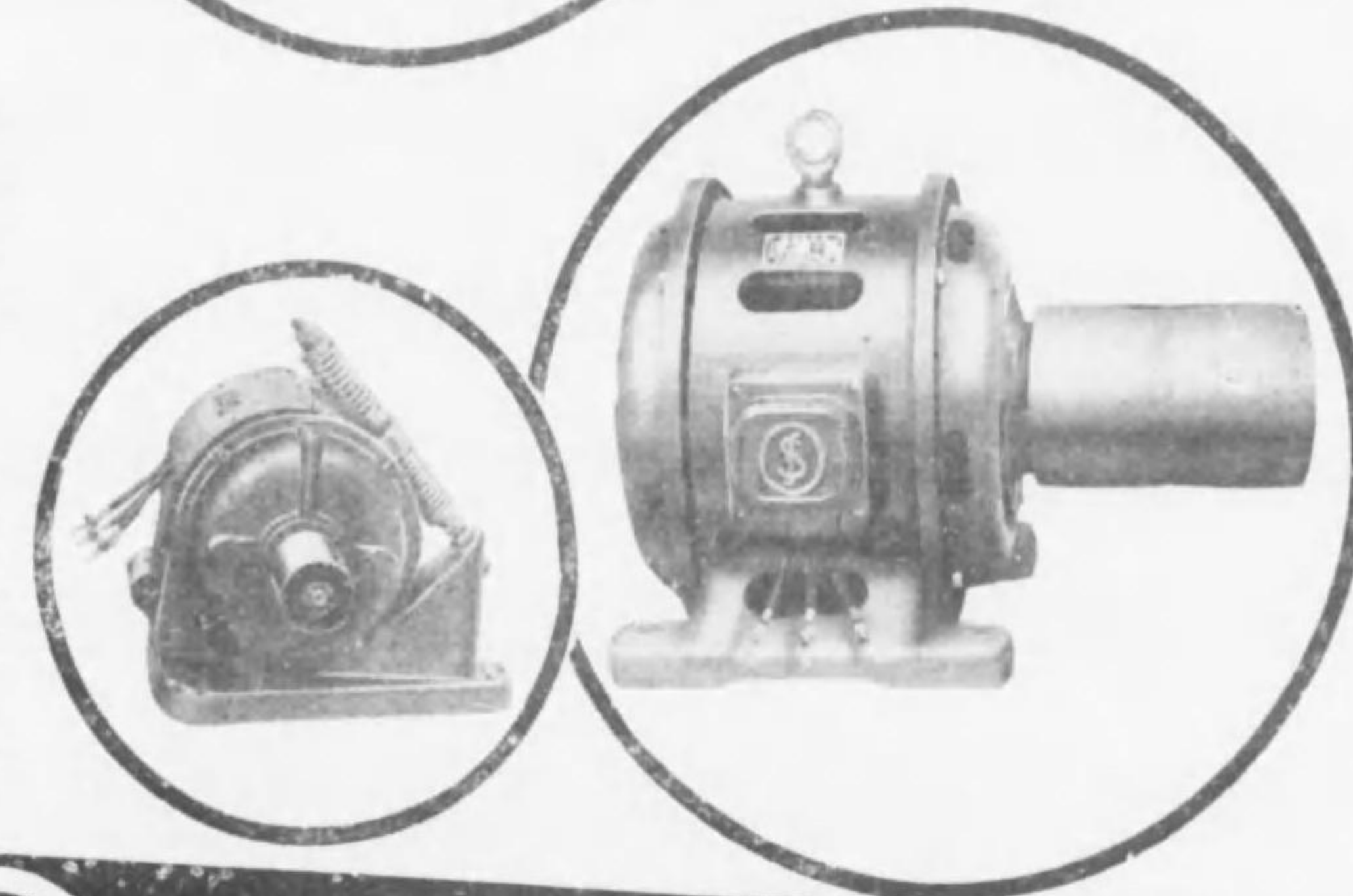
織機單獨運轉用特殊高能率電動機
