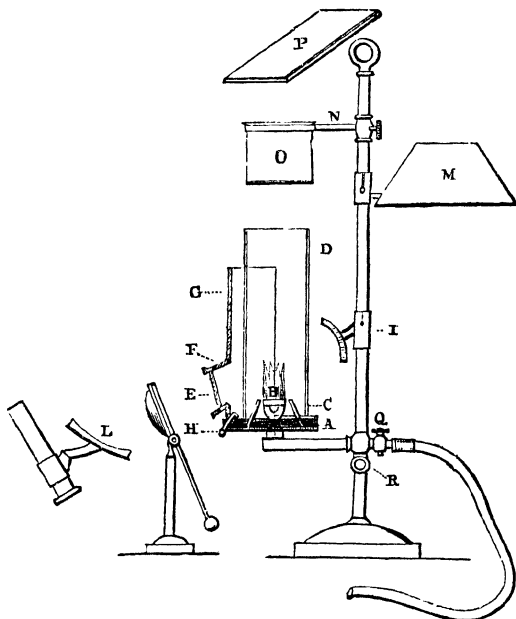
Fig. 48.—Gas-lamp, &c.
