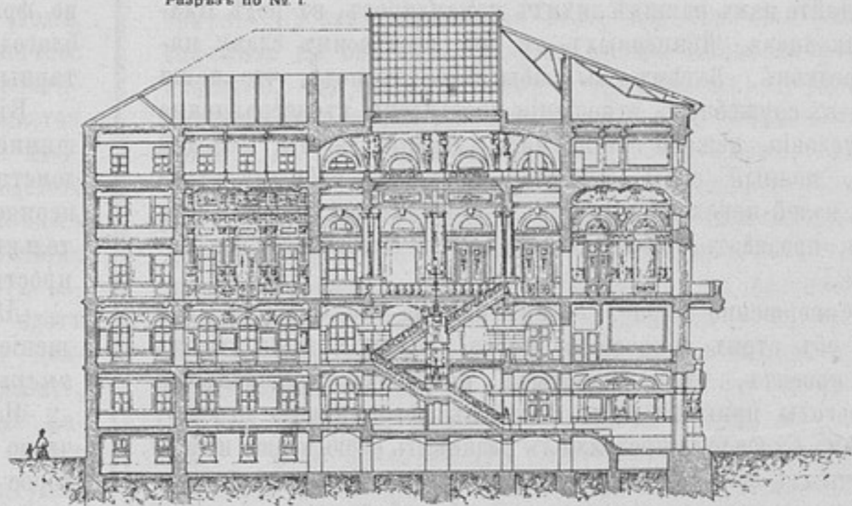
Разрѣзъ по № 1
