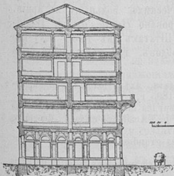
Разрѣзъ по № 3
