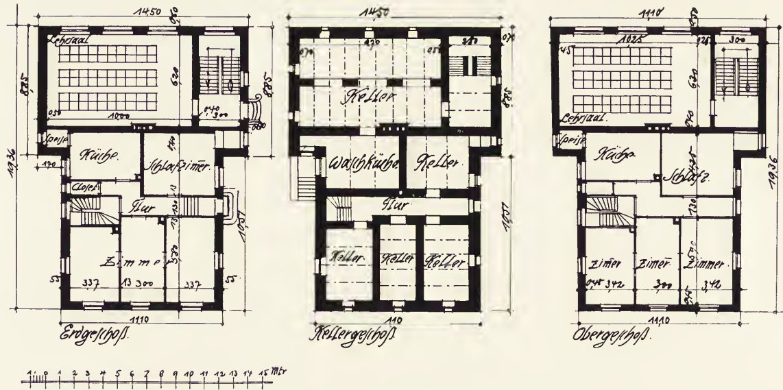
Baurat Zimmermann-Heppenheim: Grundrisse des Schulhauses in Kirchhausen
