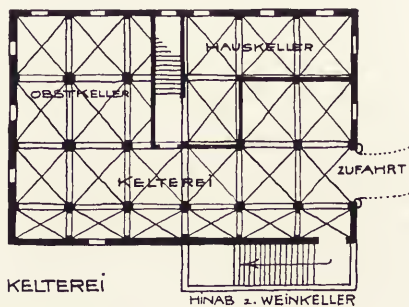
PROF. RICHARD BERNDL-MÜNCHEN Studie zu einer Kapelle, darunter Grundrisse des Weingutes in der Pfalz und des Landhauses in Solln
