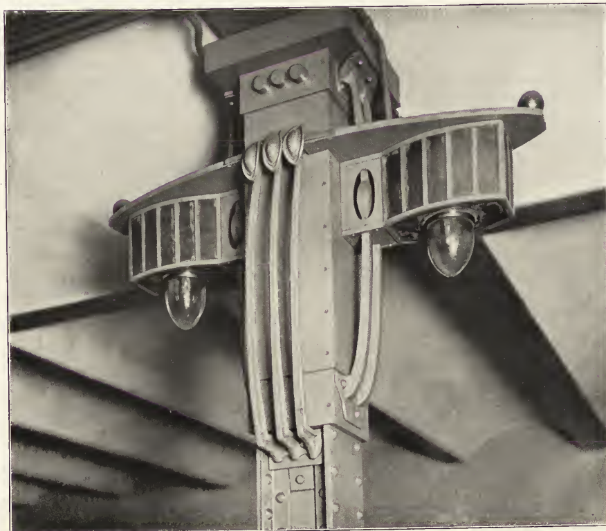
PROF. ALFRED GRENANDER-BERLIN Elektr. Hoch- und Untergrundbahn in Berlin: Stützenkopf im Bahnhof Bismarckstrasse
