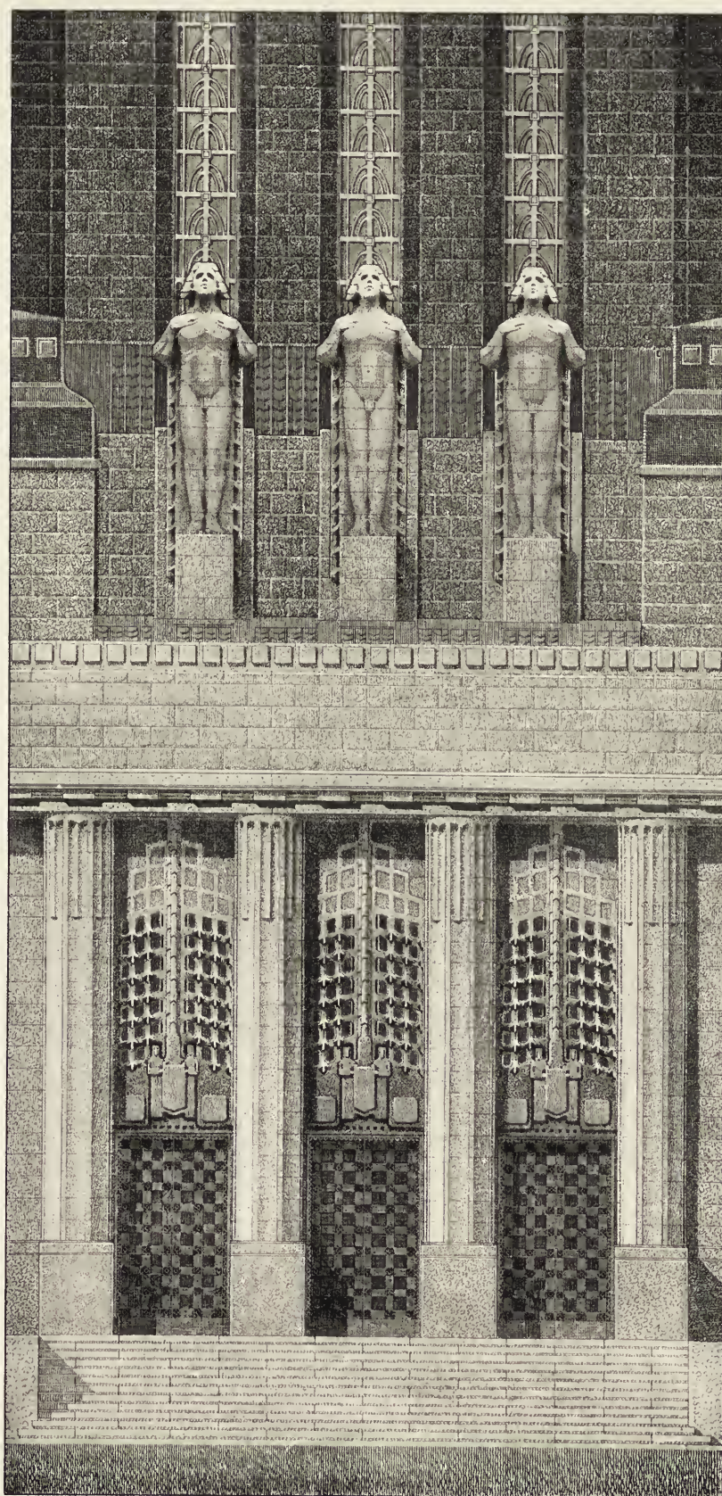
ELIEL SAARINEN-HELSINGFORS Landtaggebäude für Helsingfors: Detailstudie
