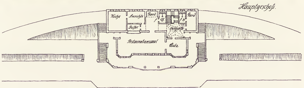
ARCHITEKT ALEXANDER HOHRATH-DRESDEN Klubhaus
