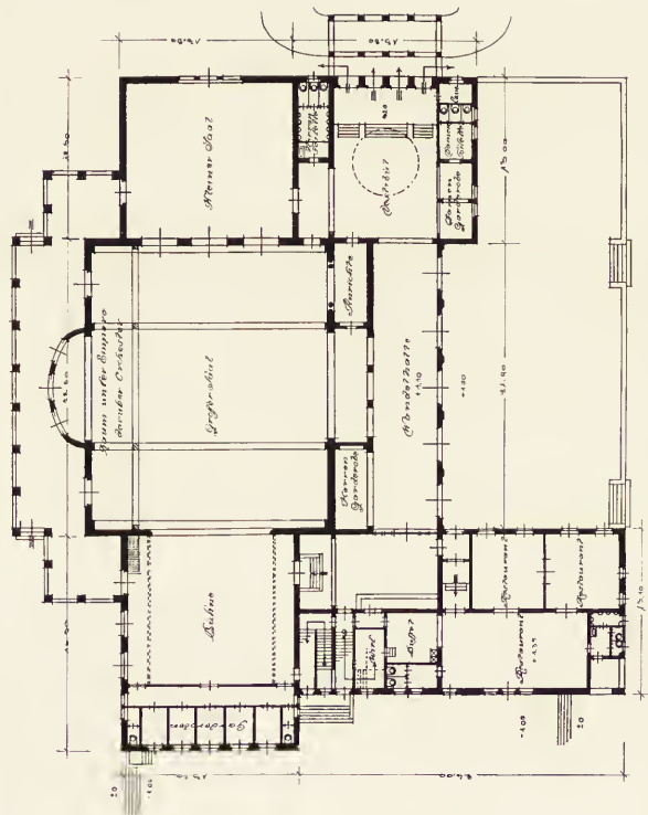
Konkurrenzentwurf für das Casino in Celle
