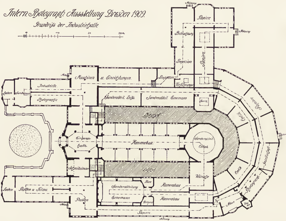
ARCHITEKT ALEXANDER HOHRATH-DRESDEN Internat. Photograph. Ausstellung Dresden 1909: Lidtbild- und Reklamewand und Grundriss der Industriehalle
