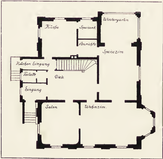
ESCH & ANKE-MANNHEIM Haus für Ludwigshafen
