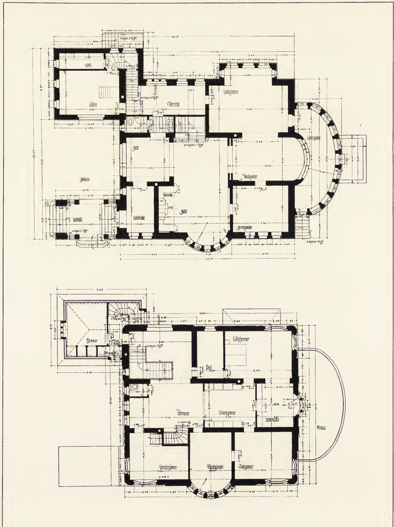
RUDOLF BITZAN-DRESDEN Wohnhaus im Riesengebirge: Grundrisse
