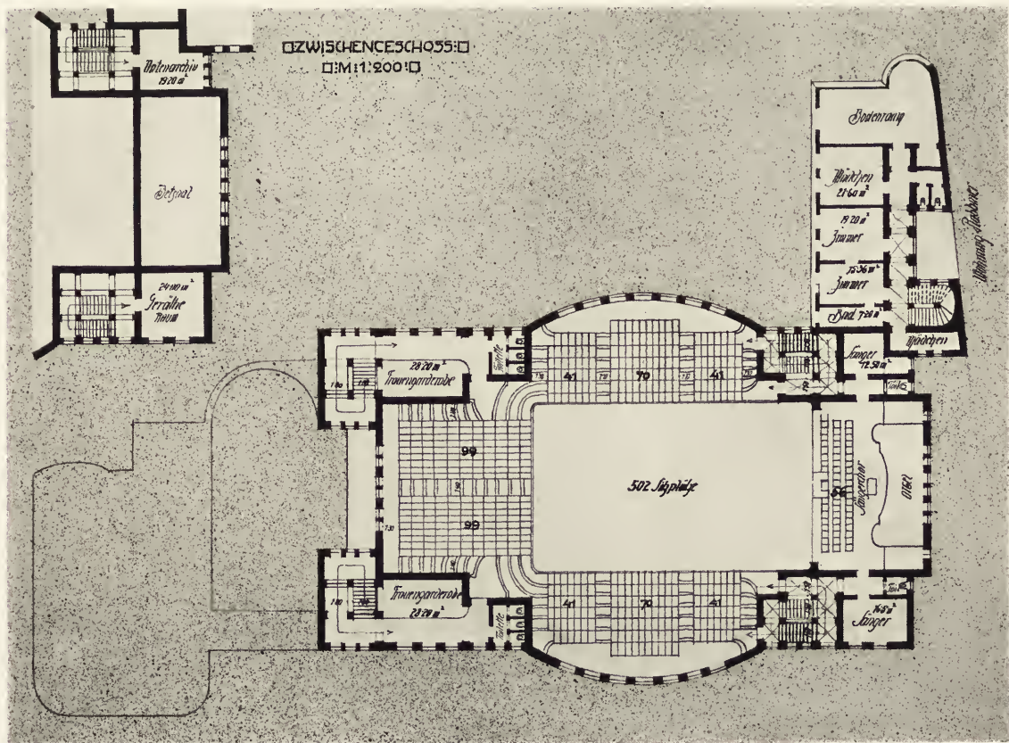
RUDOLF BITZAN-DRESDEN Wettbewerb-Entwurf zu einer Synagoge für Essen
