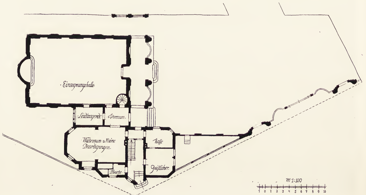
Grundriss der Eingangshalle von dem Verwaltungsgebäude auf dem Paulifriedhof
