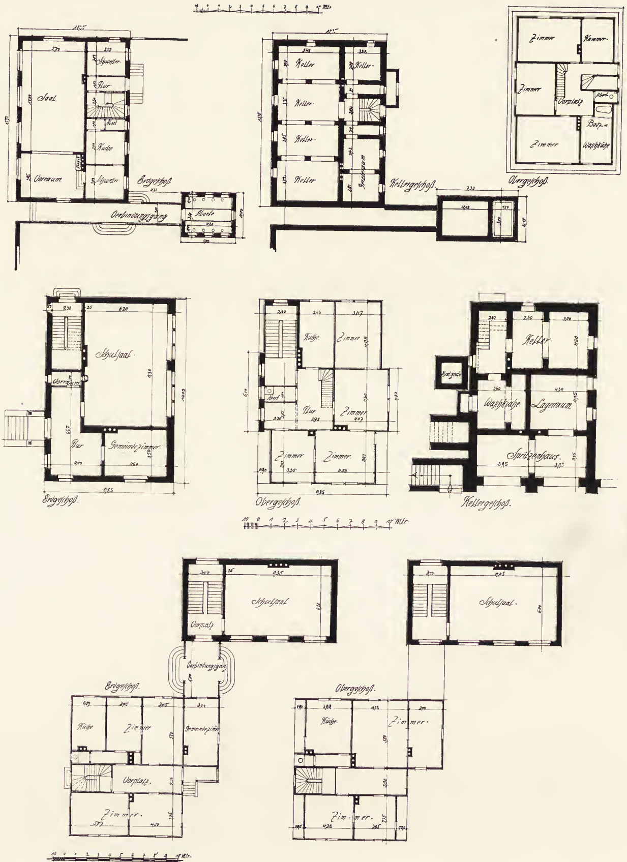
Baurat Zimmermann, Grundrisse der Kleinkinderschule in Birkenau, der Schule in Erbach und der Schule in Oberlandebach
