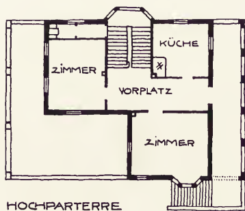
PROF. RICHARD BERNDL-MÜNCHEN Studie zu einer Kapelle, darunter Grundrisse des Weingutes in der Pfalz und des Landhauses in Solln
