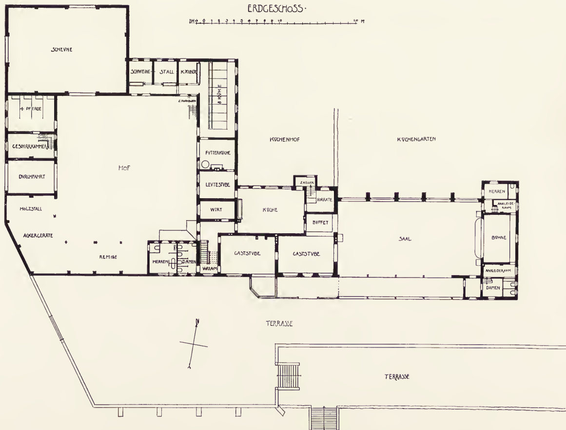
J. Mormann-Münster: Grundriss zu der Sommerwirtschaft im Münsterland
