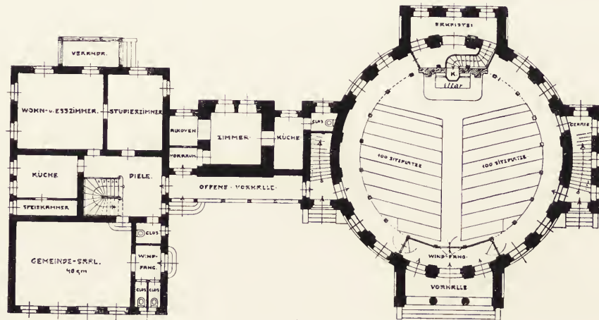
OTTO BARTNING, Grundriss der Kirche für Rottenmann
