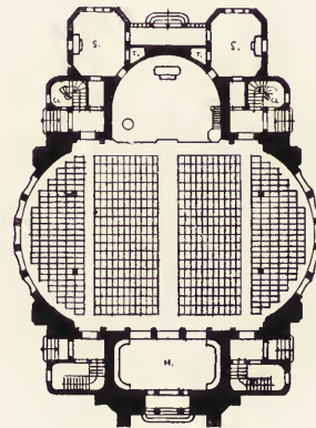
ARCHITEKT RUDOLF KOLBE, DRESDEN-LOSCHWITZ Heilandskirche für Cotta
