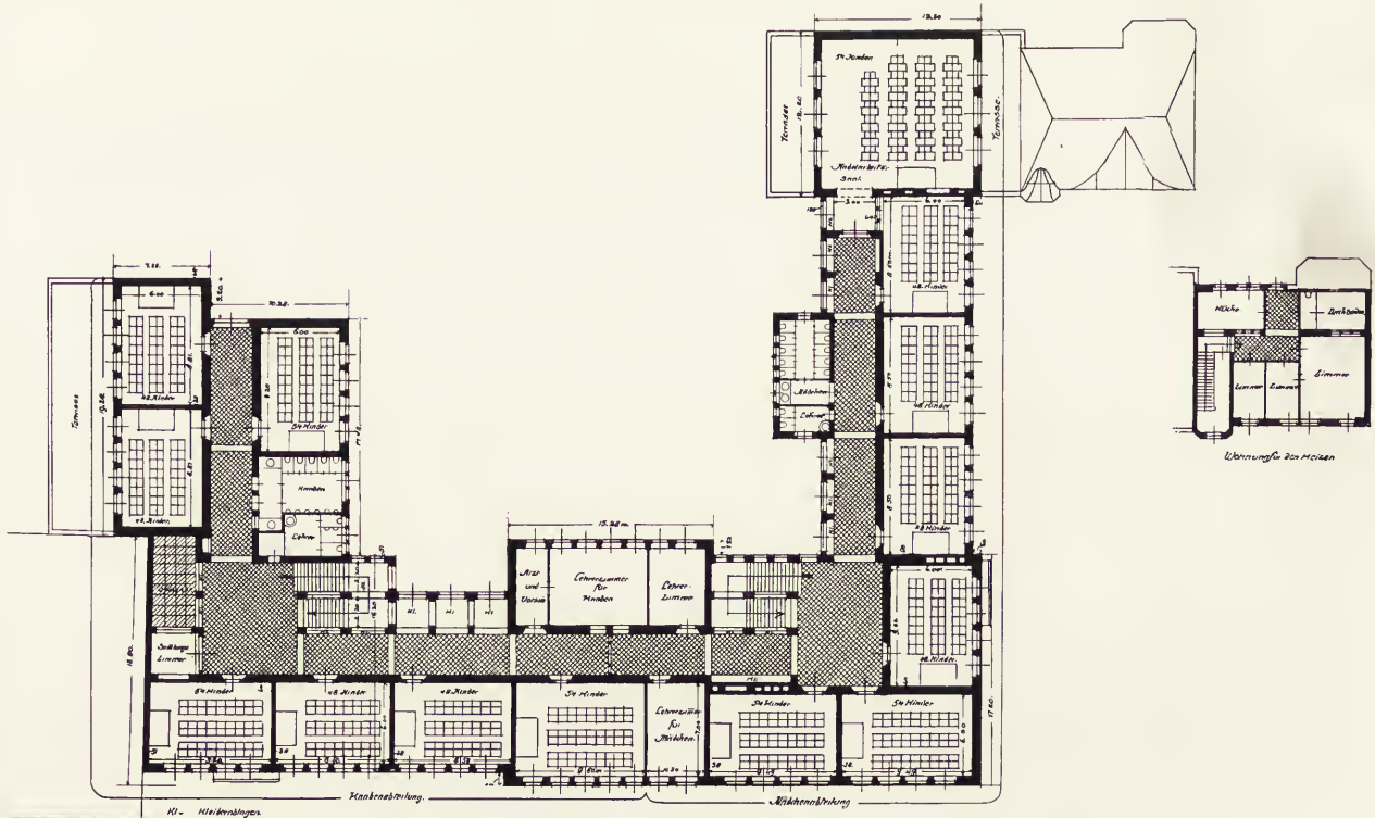
1. Obergeschoss.
