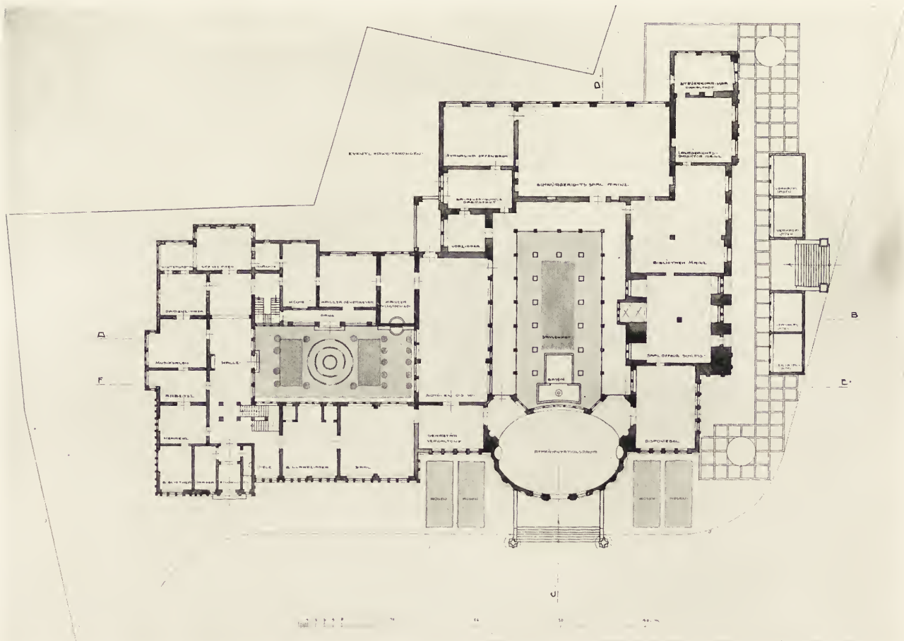
PHILIPP SCHÄFER & HANS HIRTH-DÜSSELDORF Wettbewerb-Entwurf für ein Ausstellungsgebäude (III. Preis)
