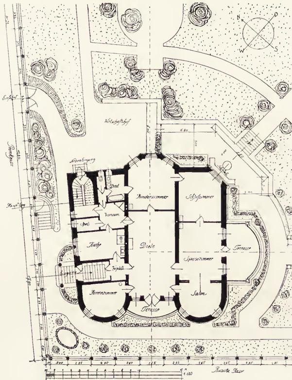
Oben: Ernst Prinz-Kiel, Grundrisse zu dem Postgebäude für Kiel-Hassel Unten: F. v. Krauss & J. Tölk-Wien, Grundrisse des Wohnhauses in Neutitschein und der Boothütte in Attersee
