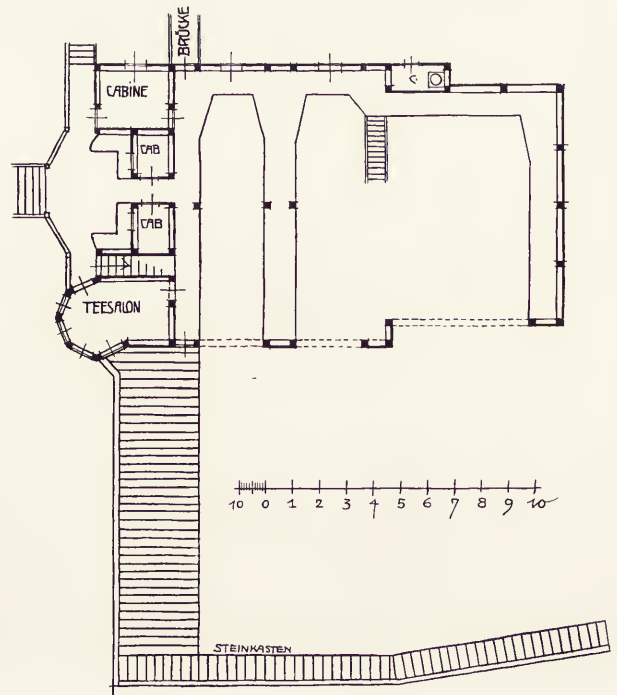
Oben: Ernst Prinz-Kiel, Grundrisse zu dem Postgebäude für Kiel-Hassel Unten: F. v. Krauss & J. Tölk-Wien, Grundrisse des Wohnhauses in Neutitschein und der Boothütte in Attersee
