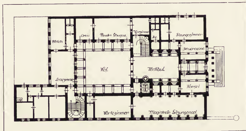
ELIEL SAARINEN-HELSINGFORS Grundriss des Stadthauses für Willmannstrand
