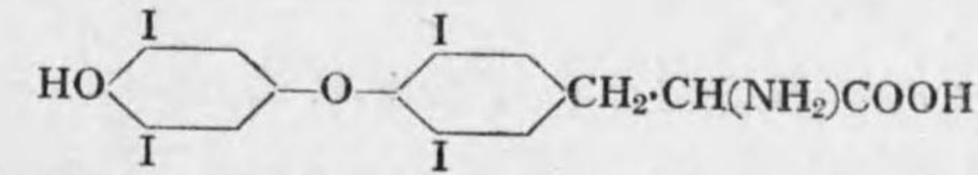
β-[3:5-Dijodo-4-(3':5'-dijodo-4'-oxyphenoxy)-phenyl]-α-Aminopropion-酸
