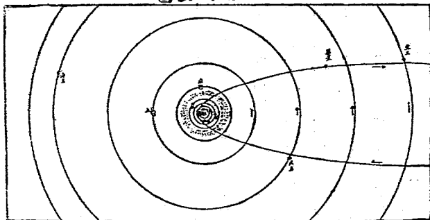
日系行星圖
