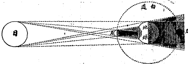
日食原理解圖
