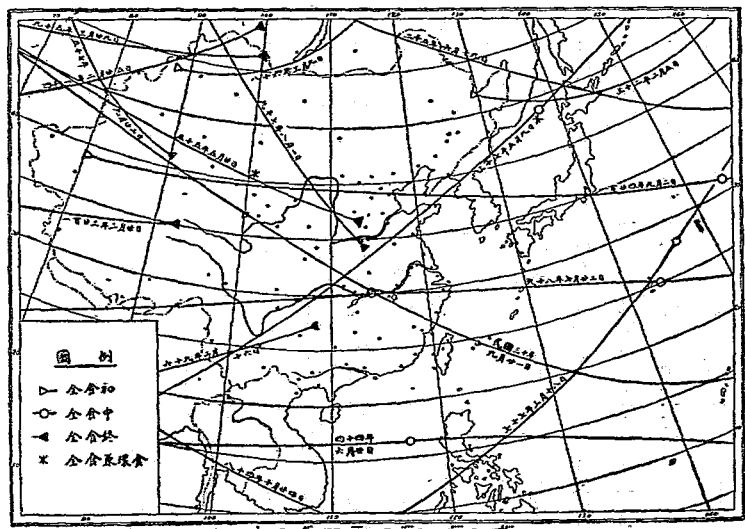
近百年內東亞日全食路徑略圖
