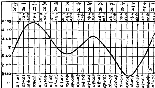
時差曲線圖
