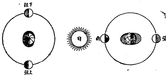
汐潮小成力分月日
