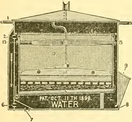
FIG. 3.—LONGITUDINAL.
