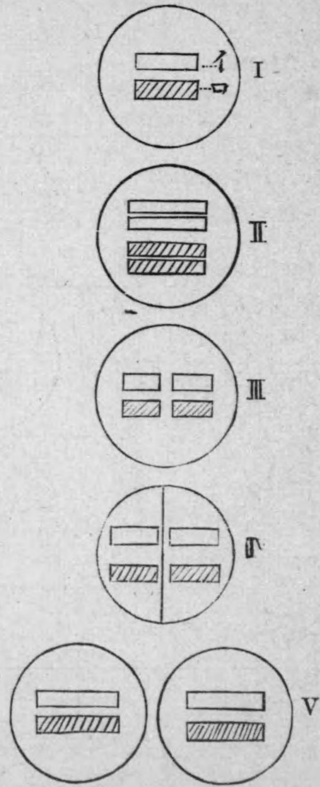
第一圖 同型核分裂の模式圖
