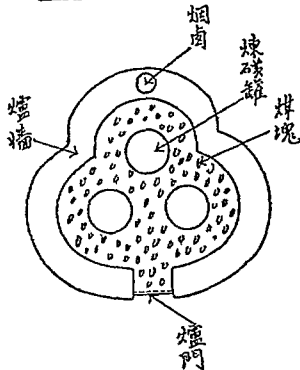
(丁) 煉爐橫切面圖
