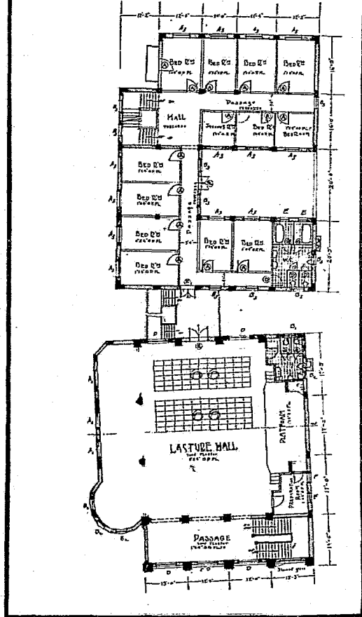
三樓構造圖
