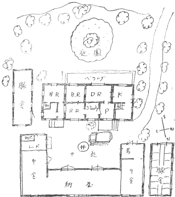
中等農家尼魯生氏之住宅及其平面圖
