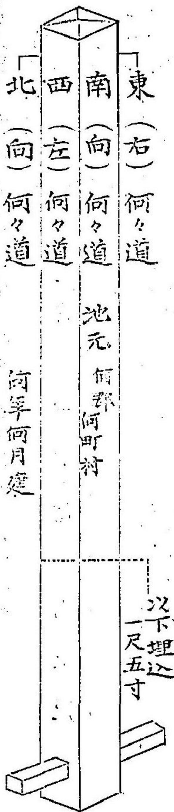
標杭雛形
