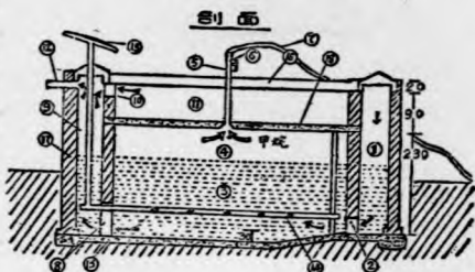
发酵池简图
