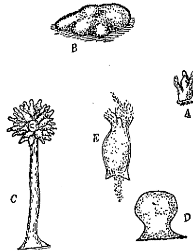
第三圖 黏質細菌之形態
