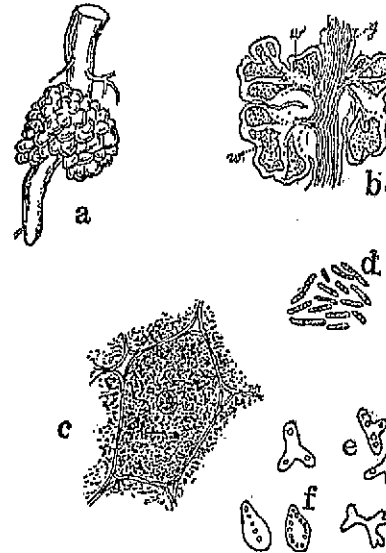
第四圖 豆科植物之根瘤菌
