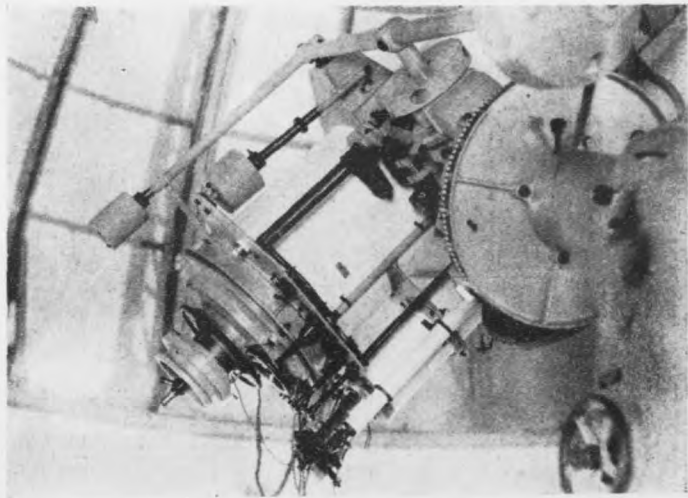
儀 道 赤 大 (圖 十 第)
