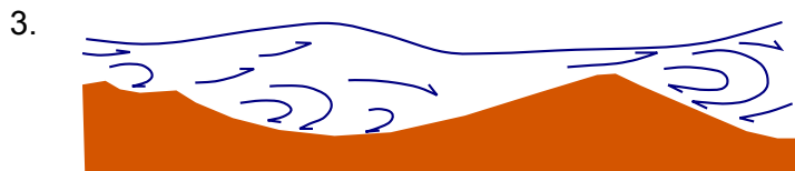
Dunes
