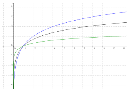
Logarithmen zu verschiedenen Basen
