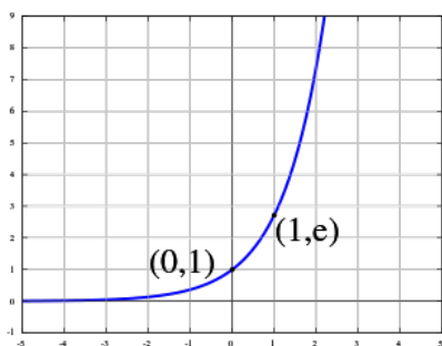
Der Graph der reellen Exponentialfunktion
