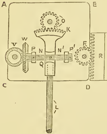
FIG. 15.—Sectional plan.
