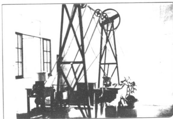
農學院新裝置之土壤試驗用機械
