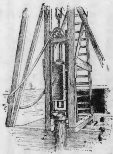
第 四 十 六 號 汽 錘 打 樁 機
