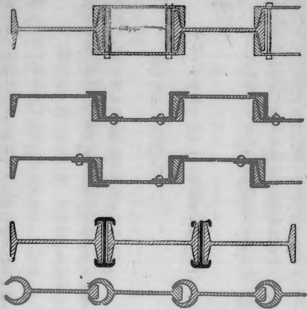
樁 放 鋼 圖 五 十 四 第
