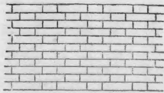
第三十九圖 法蘭德斯式磚工結合
