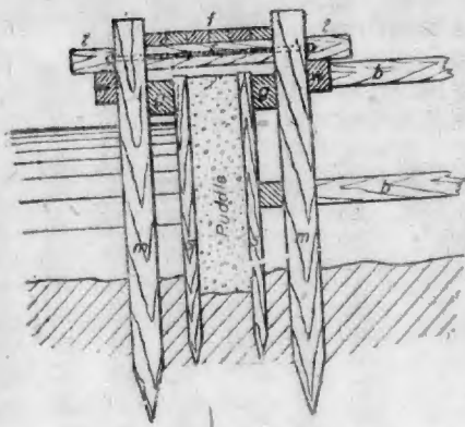
第 四 十 七 圖 土 心 牆 圍 堰
