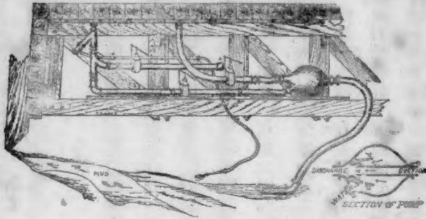
圖一十五 伊香式爛泥唧機
