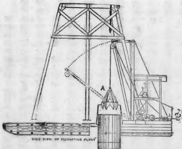
掘開筒井 圖九十四第
