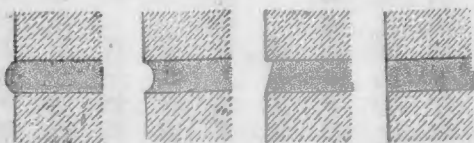
法一第 法二第 法三第 法四第 圖七十第 琢石工平縫修整法
