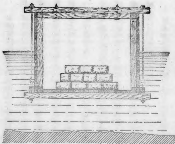
箱口敞 圖八十四第
