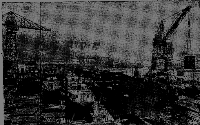
▲ 中蘇合營大連建造和修理輪船公司，幾年來對我國航運事業的發展起了巨大的作用。根據中蘇會談公報的規定，不久即將完全成為我國的國營企業了。這是工人們運用蘇聯分型造船法的先進經驗造船的情形。劉培廣攝
