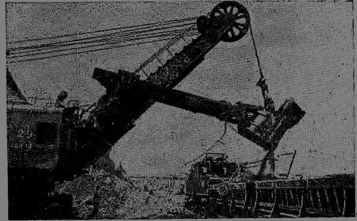
▲ 蘇聯政府以現代化的機械設備來裝備我國的工業。阜新海州露天煤礦使用蘇聯電鍍剝土機，一小時能剝土三立方公尺土。這是某電鍍小組在剝土機上工作的情形。賈承濱攝
