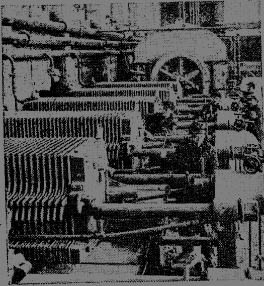
△國營太原鋼鐵廠電爐煉鋼部擴建的幾部電爐，其中某部電爐已開始通電煉鋼。擴建的電爐都投入生產後，該部今年的產量將比一九五四年增長二點五倍。這是新投入生產的某部電爐正在出鋼。(周樹銘攝)
