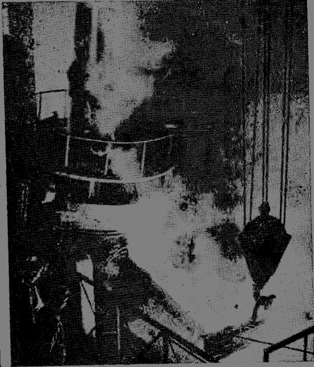
△國營太原鋼鐵廠電爐煉鋼部擴建的幾部電爐，其中某部電爐已開始通電煉鋼。擴建的電爐都投入生產後，該部今年的產量將比一九五四年增長二點五倍。這是新投入生產的某部電爐正在出鋼。(周樹銘攝)
