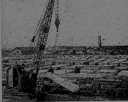
△第一汽車製造廠今年的工程已開始全面施工，施工所需的各種材料，源源運往現場。上圖：第一汽車製造廠鋼筋預製工廠生產的大批構件，正往施工現場運送，供施工需要。左圖：第一汽車製造廠最後開工的一座生產廠房——整車車間，正動工興建。(雷印攝)
