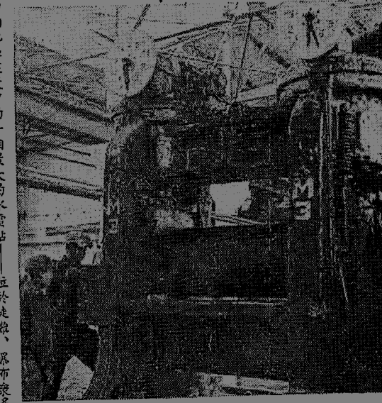
△在龍崗江省佳木斯市建設的我國第一座現代化的為造紙工業服務的佳木斯鋼網廠，不久就要投入生產。圖為安裝工人正在調整該廠重要設備之一——雙龍壓延機，準備試運行。(王純德攝)(本報並刊照片全係新華社攝)
