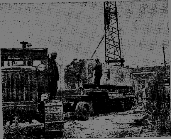
△今年，鑄鋼在土方、運輸、起重及製造混凝土的工作中，機械化施工的工作量比去年增加兩倍左右。機械化、工廠化施工的採用，對今年鑄鋼建設工程的勝利完成將起重要作用。上圖：十噸重的混凝土預製構件，已在工廠製成，正裝上拖車準備運往工地。右圖：在化工工地，塔式吊車正將鋼筋、木料吊到數十公尺高的建築物上，供在高空作業的工人使用。(楊禮門攝)
