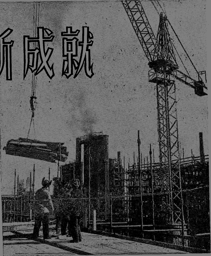
△今年，鑄鋼在土方、運輸、起重及製造混凝土的工作中，機械化施工的工作量比去年增加兩倍左右。機械化、工廠化施工的採用，對今年鑄鋼建設工程的勝利完成將起重要作用。上圖：十噸重的混凝土預製構件，已在工廠製成，正裝上拖車準備運往工地。右圖：在化工工地，塔式吊車正將鋼筋、木料吊到數十公尺高的建築物上，供在高空作業的工人使用。(楊禮門攝)
