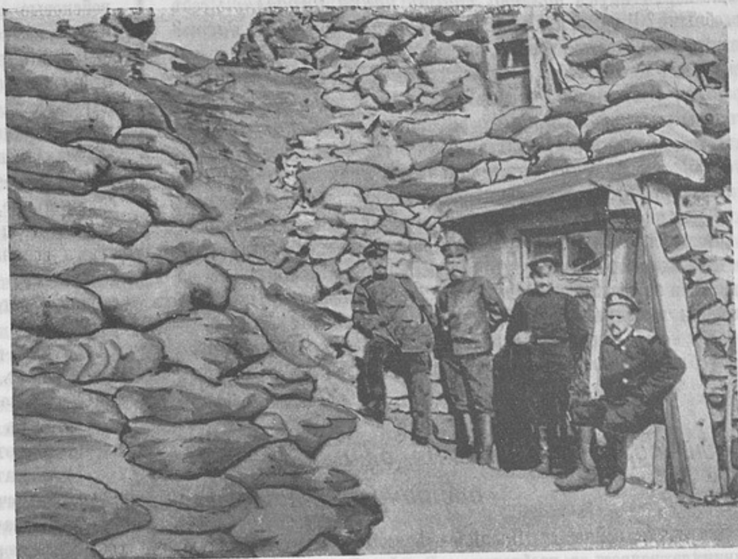
Блиндажи на Орлиномъ гнѣздѣ. (Изъ книги «Оборона Портъ-Артура» см. «Библ.»).
