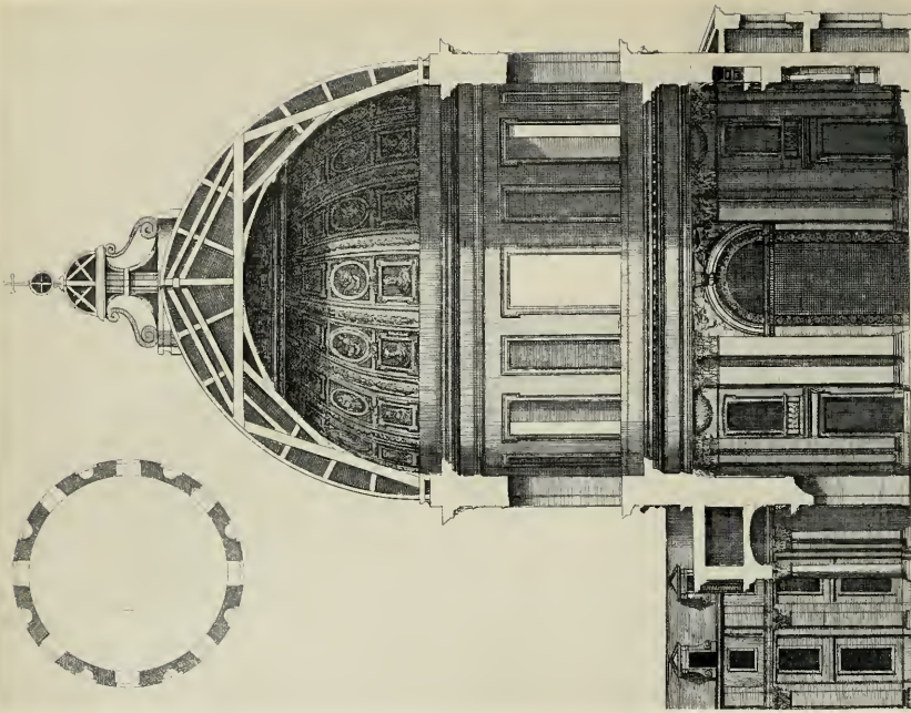
Section de l'Église des Religieuses de l'Assomption rue et Honneur du duc de Nemours, par M. Errard
