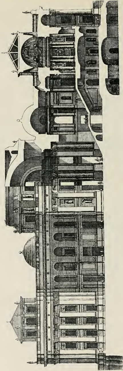
ESLEVATION DE LA MOITIE DE LA FASCE DU BATIMENT ENSEMBLE LA VEVE ET PROFIL DU VESTIBULE ESCALIER ET DE S' DEDANS DES SAILONS ET PORCHES ALLANS AV PARTERRE ET OFFICES AV DEDANS .
