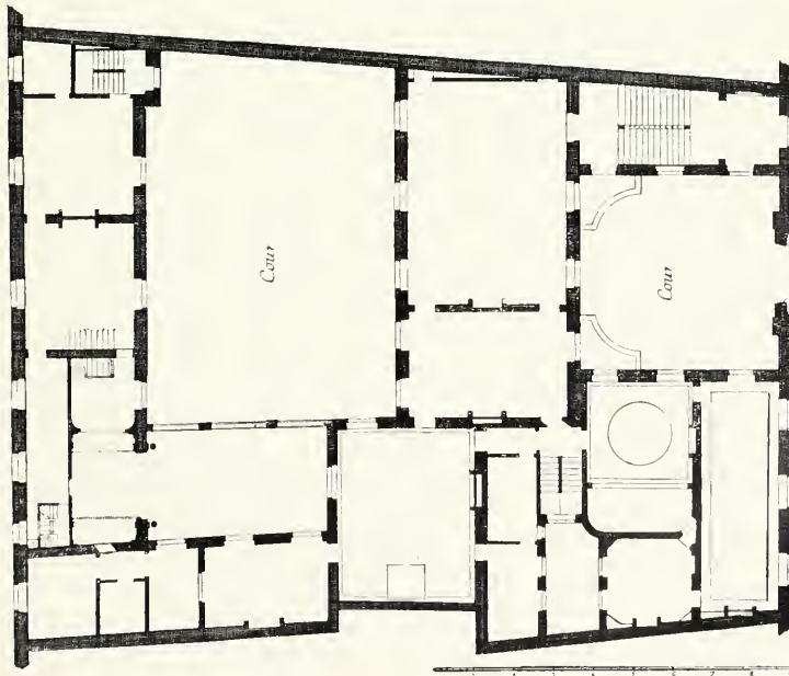
Plan du premier étage de l'hostel de Bisceuil
