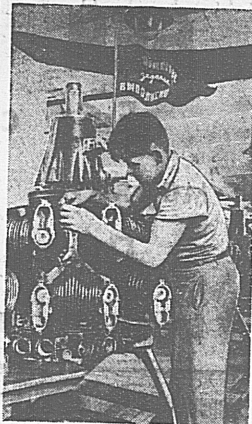
По несколько авиационных моторов в сутки сверх плана дает цех окислительной сборки моторов...
