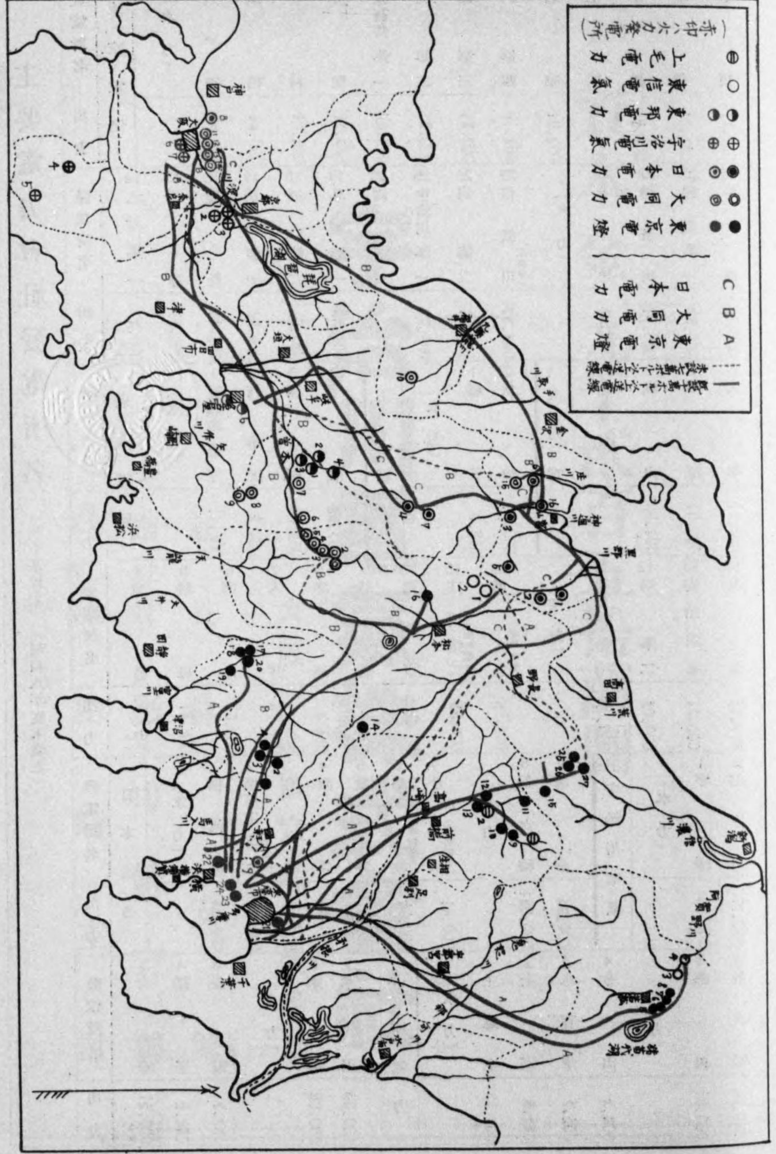
本州中部十萬ホリ以上送電線路圖
