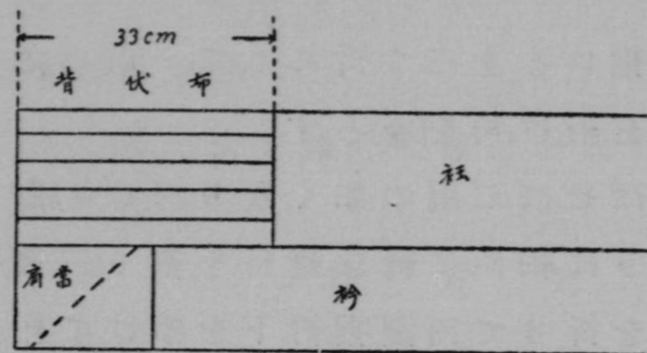
背伏布及び衿肩當の裁方
