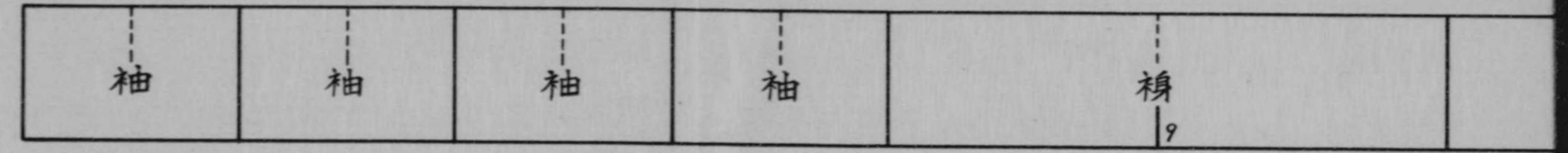
第五圖(2)無双袖別衿仕立裁方 (總用布 1180cm 内外) 一反
