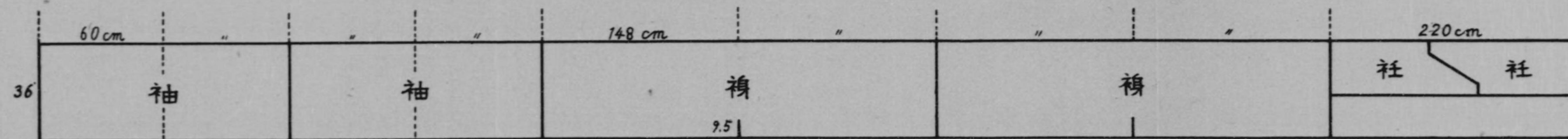
第三圖 鉤衤裁方 (總用布 1100cm)
