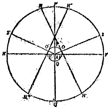
第九圖 出沒現象的說明
