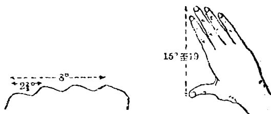
第十二圖 角度的估計方法
