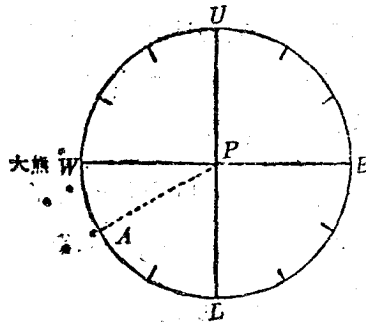
第四十四圖 大熊座 \alpha 星的利用(二)
