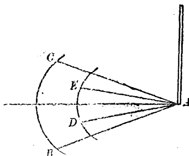
第二十二圖 用太陽求真南北方向
