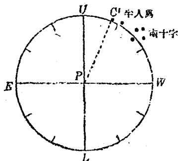
第四十八圖 半人馬座 \alpha 型的利用
