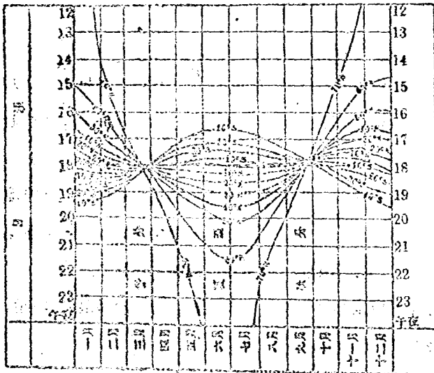
第二十圖 太陽出沒時間 已經加上時差的訂正。若求極高時，應將本表總數在本時區區鐘數子 午區的間數乘多少度，每度加減四分，圓周度減。圓周度乘訂正。
