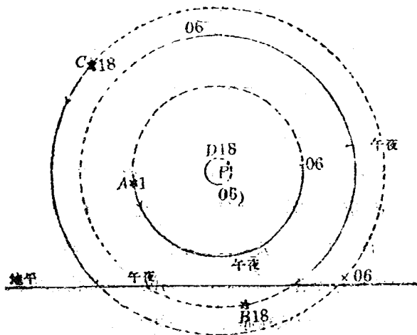
第七圖 星辰的翻動(一)
