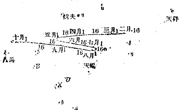
第六圖 一九二二年火星的逆行路
