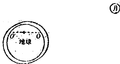
第四十圖 高潮的發生
