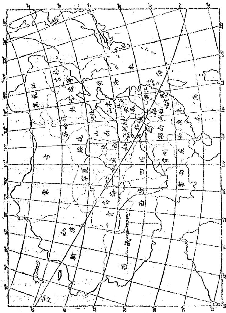
第三十七圖 民國三十年九月二十一日我國風況之全圖。
