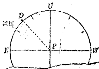
第四十九圖 波江座 \alpha 星的利用
