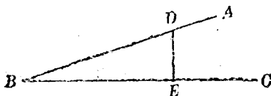
第十五圖 角的正切
