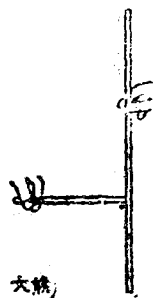
第四十六圖 大熊座 \alpha 星位置的決定
