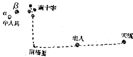
第四圖 南極星的圖說
