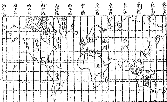
第十七圖 世界標準時區圖
