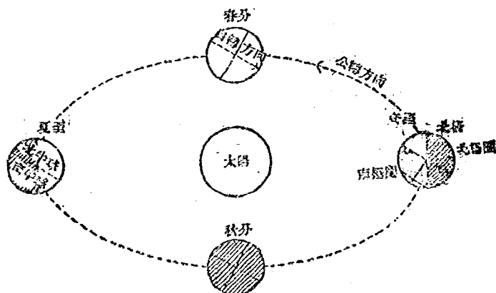
第十九圖 四季地球的位置
