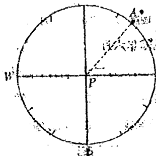
第四十五圖 太陽在赤道上(三)
