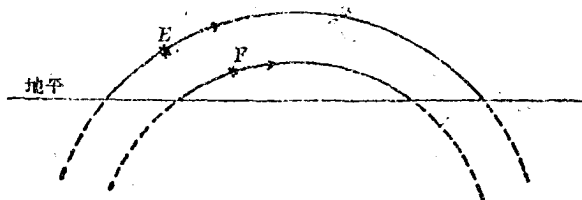
第八圖 星辰的視點(二)
