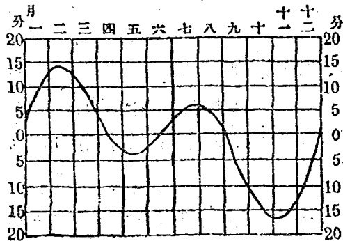
第十六圖 時差
