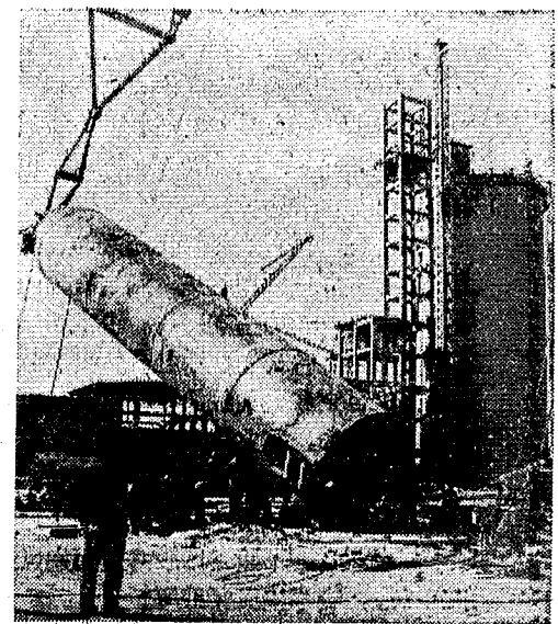
在岳阳化肥厂工地上，第四化工建设公司一处起重工人用单扒杆吊装的重量三百一十八吨的氨合成塔。本报通讯员摄
