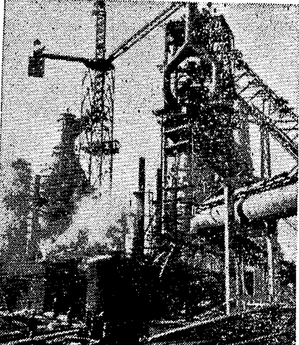
這座十號高爐是鞍鋼在兩年內建成的。圖為十號高爐出鐵。
