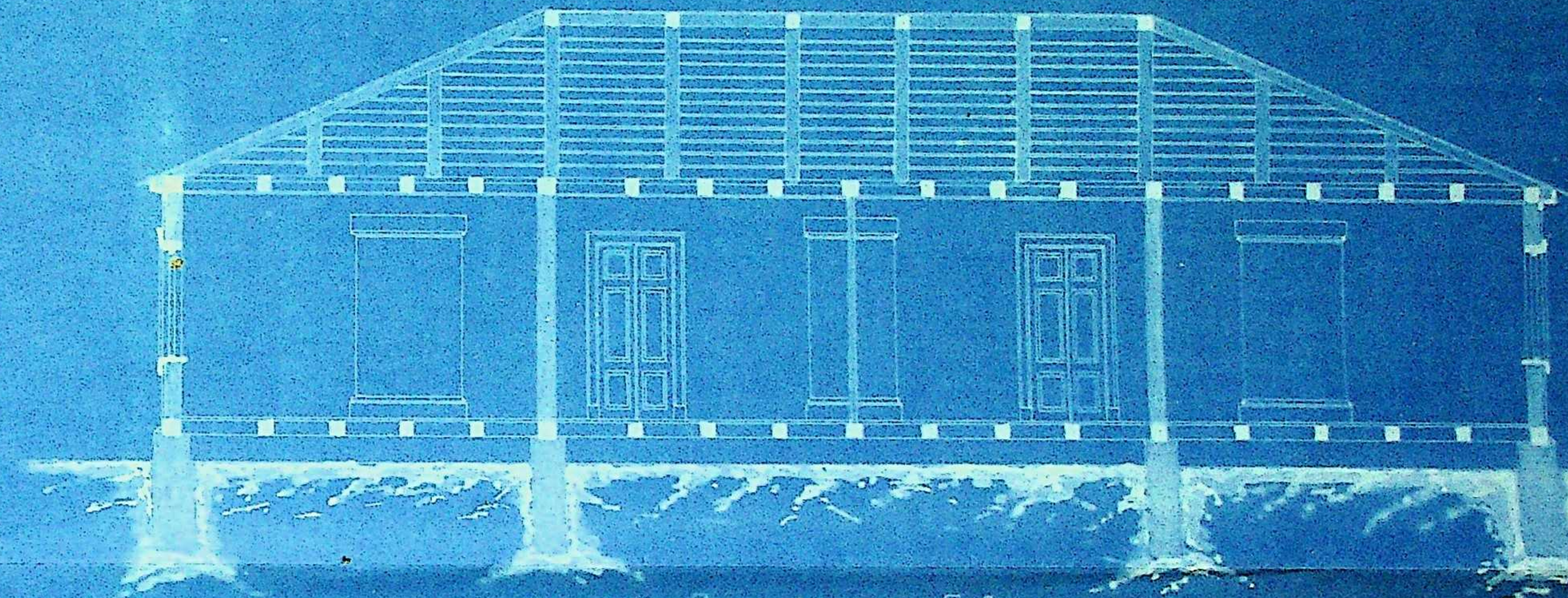
Разрѣзъ по СД
