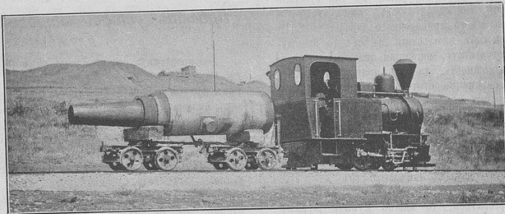
Передвиженіе паровозомъ въ 9 тон. 9-ти дм. берегового орудія на тельжкахъ образца 1895 года, колѣя 75 см. (къ рецензій «Крѣпости и крѣпостныя желѣзныя дороги»).
