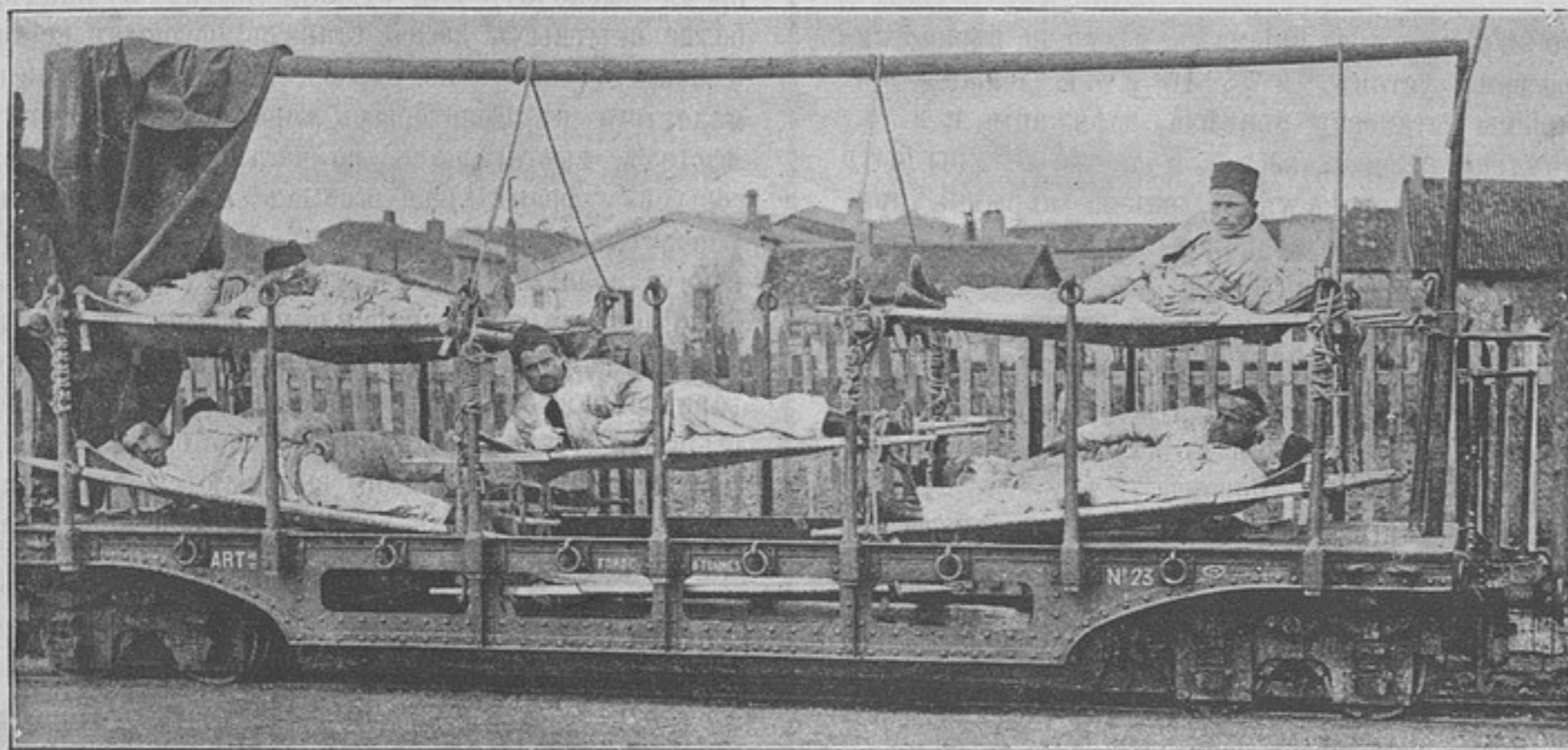
Приспособленія для перевозки раненыхъ въ вагонетахъ на 60 см. колеѣ (къ рецензій «Крѣпости и крѣпостныя желѣзныя дороги»).
